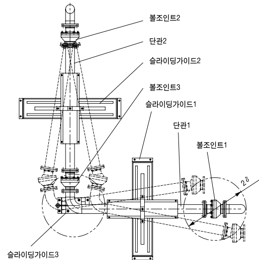
▶ 구조도
