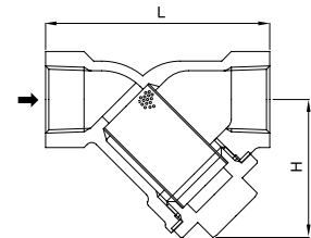
YKY-5B
