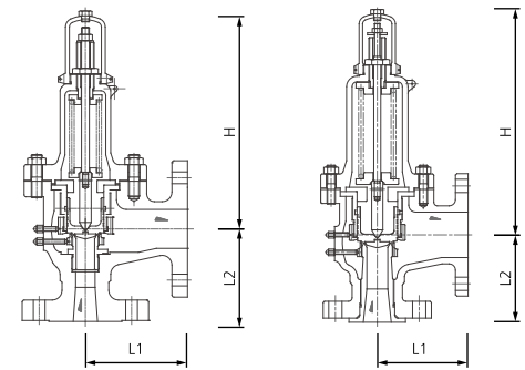
YRV-1형
