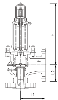
YSF-4형
