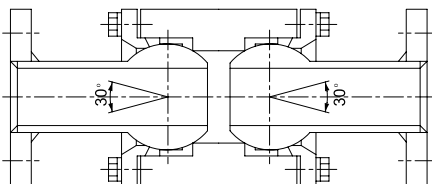
▶ 구조도
