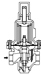
파일럿 감압밸브
