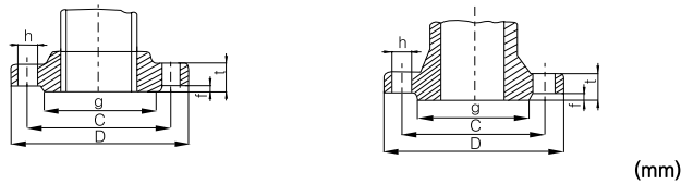
16kgf/cm 2 관 플랜지의 기준치수
