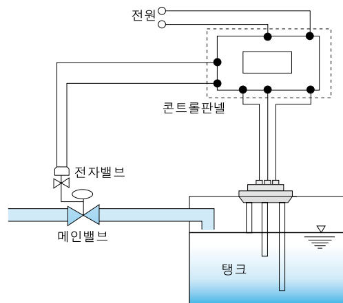
[그림 2] 전자밸브접속회로도
