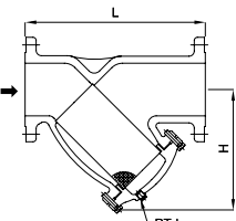
YKY-2 65~450A
