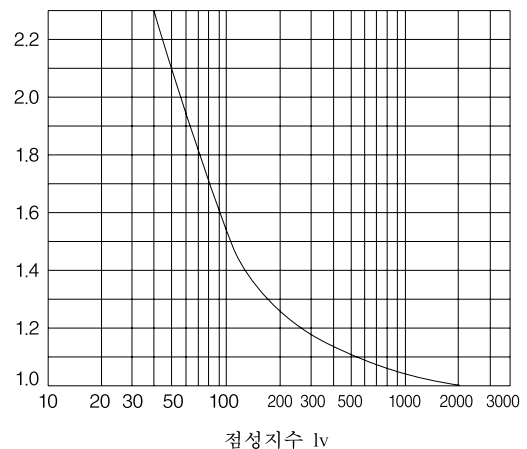
점성지수 I v -C v 보정 계수 K 관계도표
