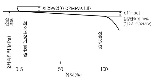
유량 특성도
