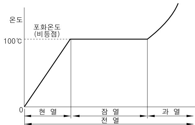
》 그림2. 열량곡선
