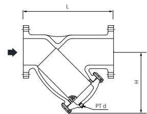
YKY-12
