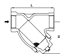
YKY-1 25~50A
