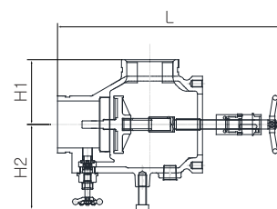
YCC-2A(20K)
