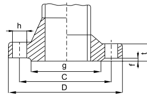
40kgf/cm 2 관 플랜지의 기준치수
