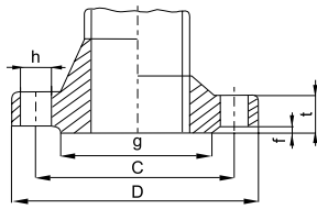
30kgf/cm 2 관 플랜지의 기준치수
