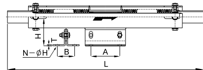
YBJ-4S형
