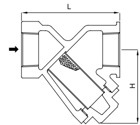
YKY-5B
