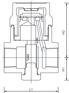
YSP-2형
