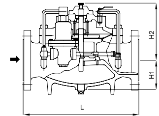
주밸브
