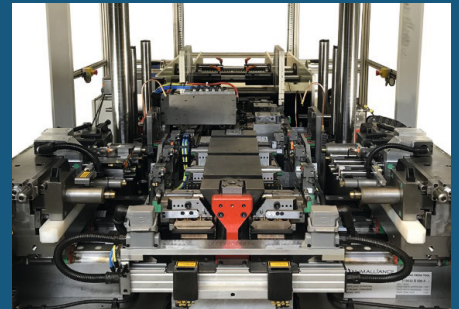
Press die
