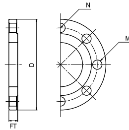
JIS RF FLANGE
