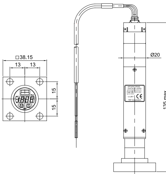
■ 15PT1-2W-***R/G-**
