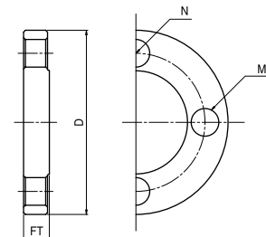
JIS BLIND FLANGE
