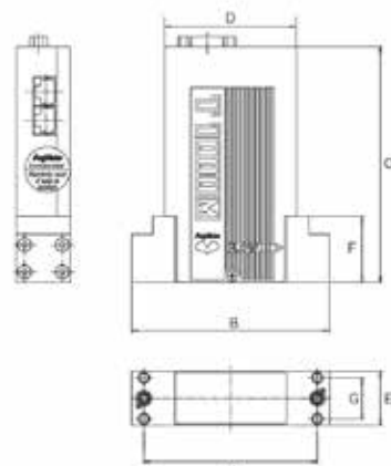
IGS Type
