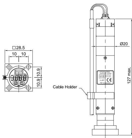
■ 11PT1-2W-***R/G-**
