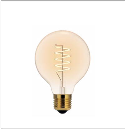
필라멘트 G80 W/C 60W / 2200K Size Ø80 x H119 mm Box(EA) 30 EA
