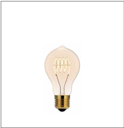
필라멘트 A60 W/C 40W / 2200K Size Ø60 x H113 mm Box(EA) 30 EA
