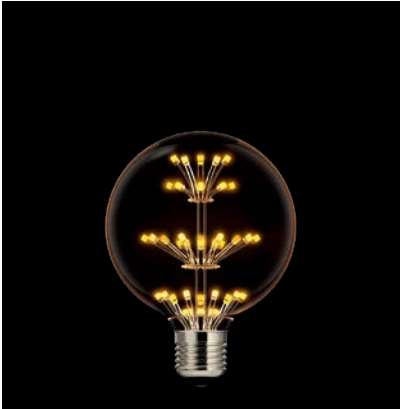
엘디자인 G95 W/C 2W / 2200K Size Ø95 x H132 mm Box(EA) 30 EA
