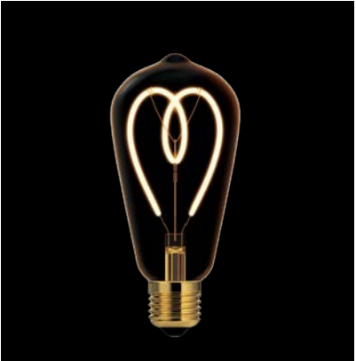
롱 하트 COB ST64 W/C 3W / 2200K Size Ø64 x H136 mm Box(EA) 30 EA
