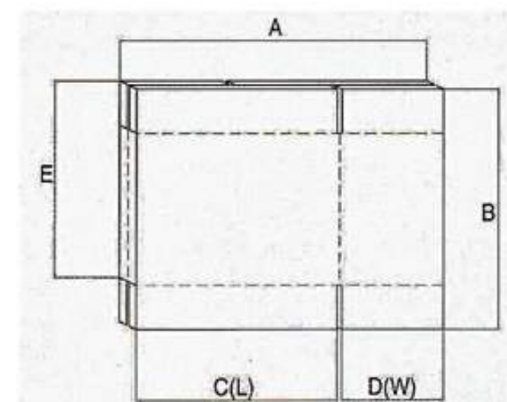
반대형 박스(OPPOSITE)
