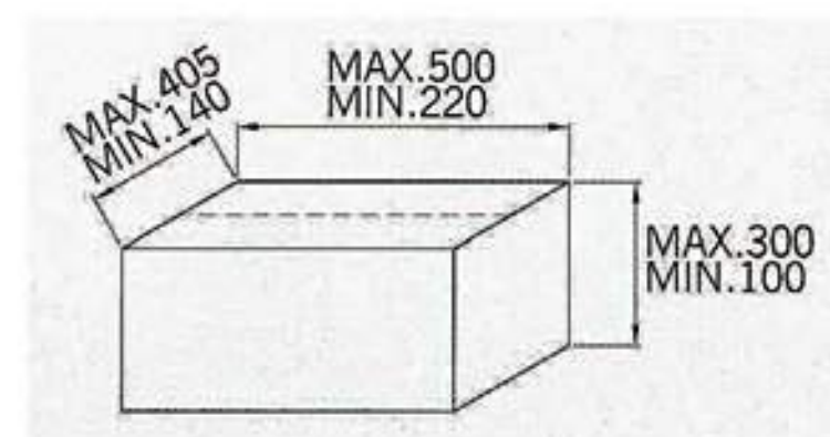
제함박스의 크기(MM)
