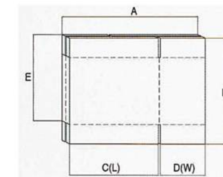
반대형 박스(OPPOSITE)
