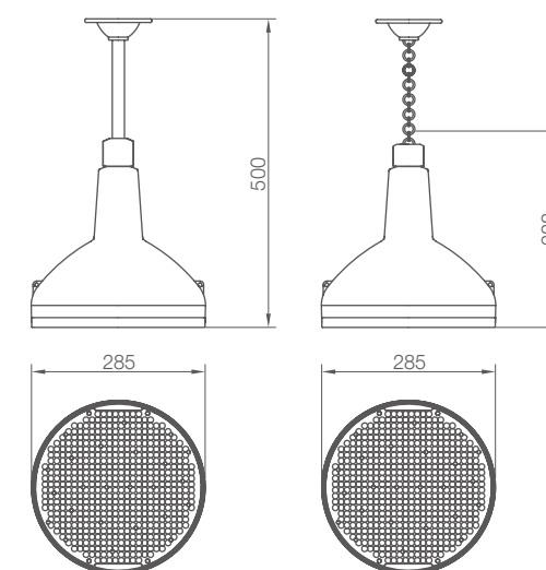
Pipe Pendant Type
