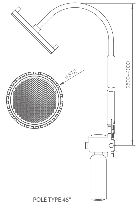
POLE TYPE 45°
