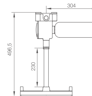
PENDANT TYPE
