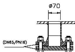
Gegenlager DF50 Seite 6 / Kapitel 6 Opposite support DF50 Page 6 / Chapter 6
