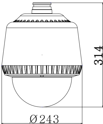
▲ FW8706-HNP 2메가픽셀 PTZ 카메라
