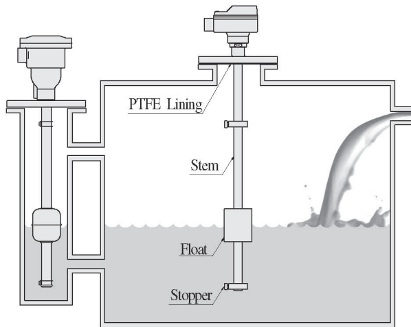
Fig.3 Sensor의 취부방법
