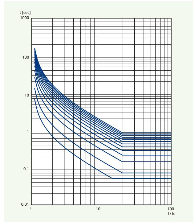
IEC-VI:Very Inverse Time
