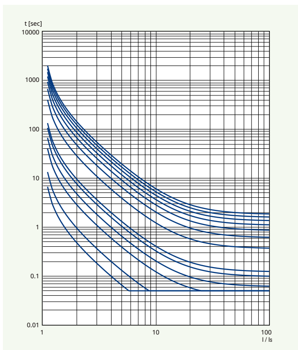
IEEE-EI:Extreme Inverse Time)
