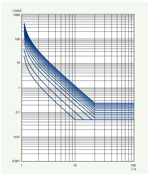
IEC-EI:Extremely Inverse Time
