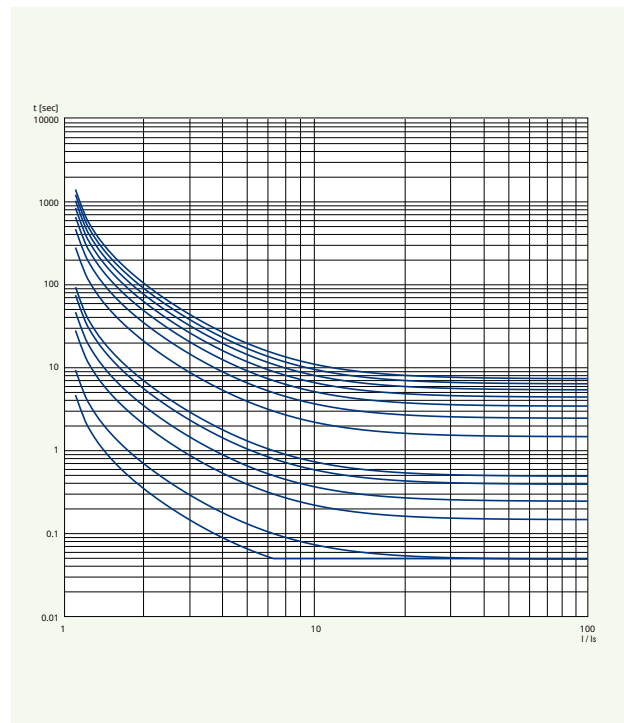
IEEE-VI:Very Inverse Time)
