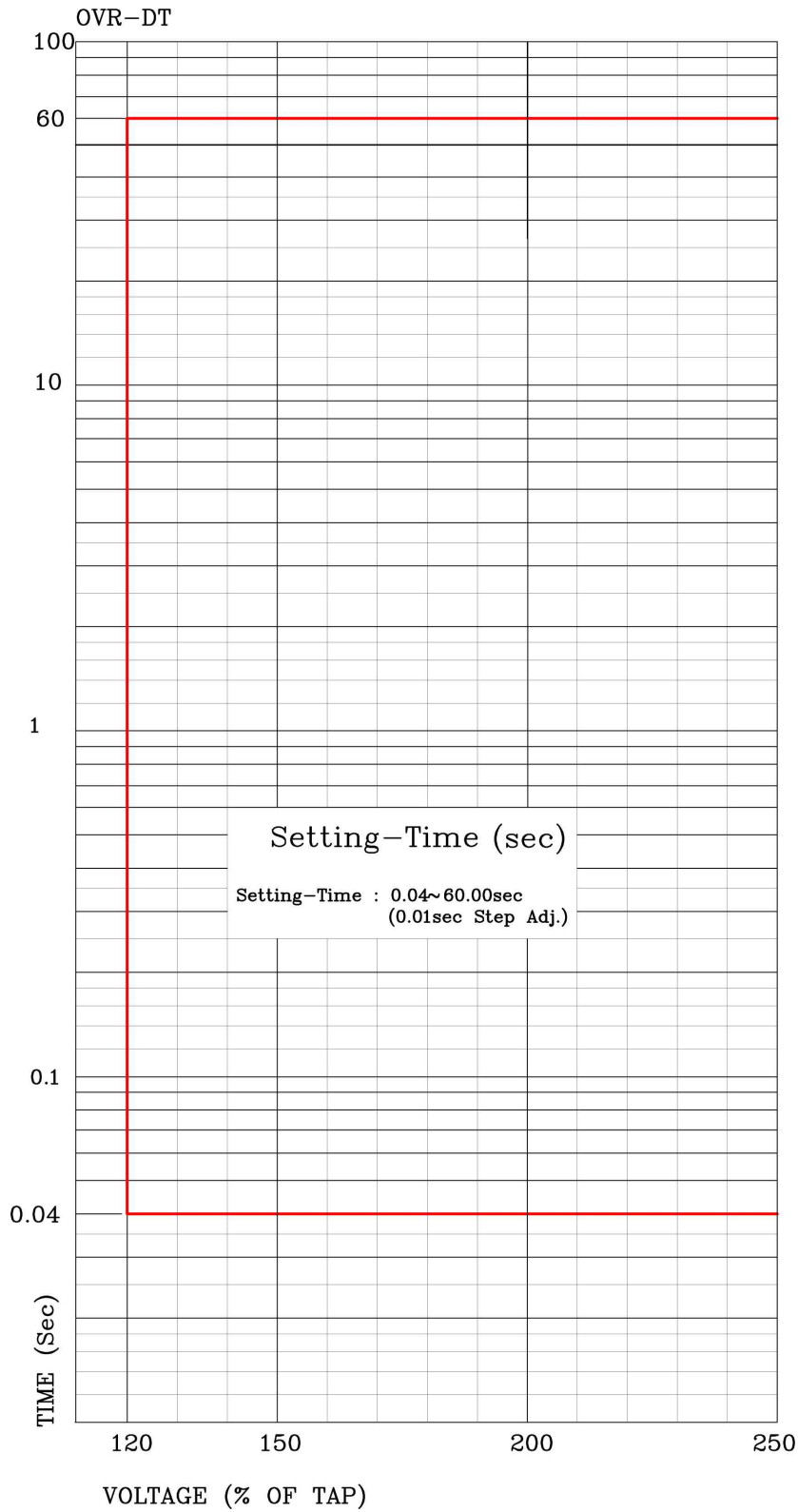
【부도 18】 과전압 요소 정한시 특성 곡선
