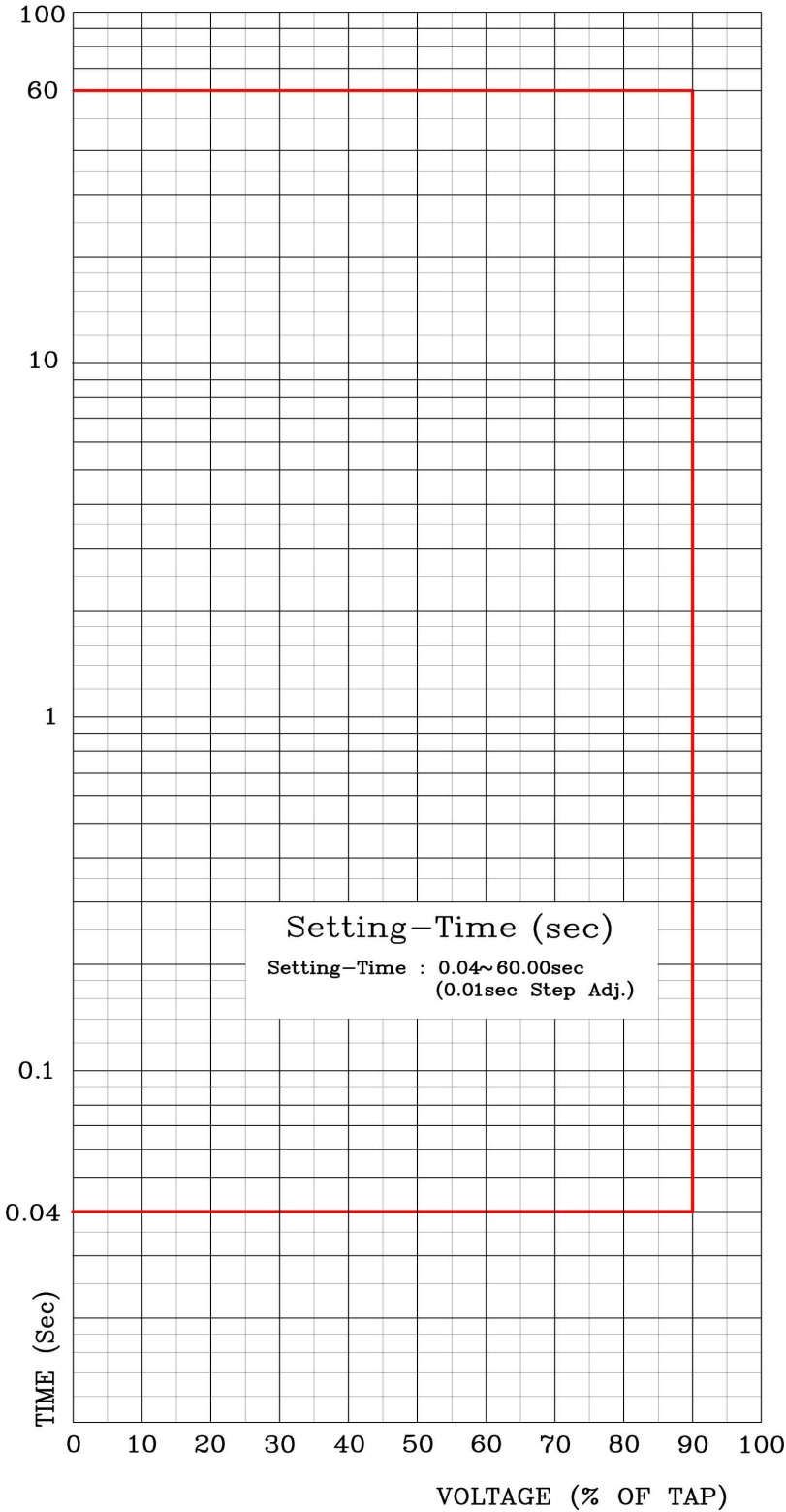
【부도 20】 저전압 요소 정한시 특성 곡선 UVR-DT
