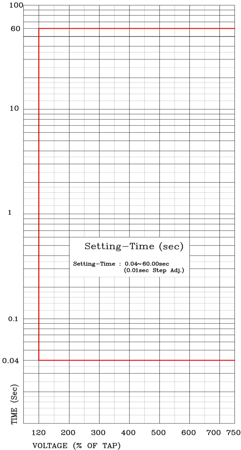
【부도 22】 지락 과전압 요소 정한시 특성 곡선 OVGR-DT
