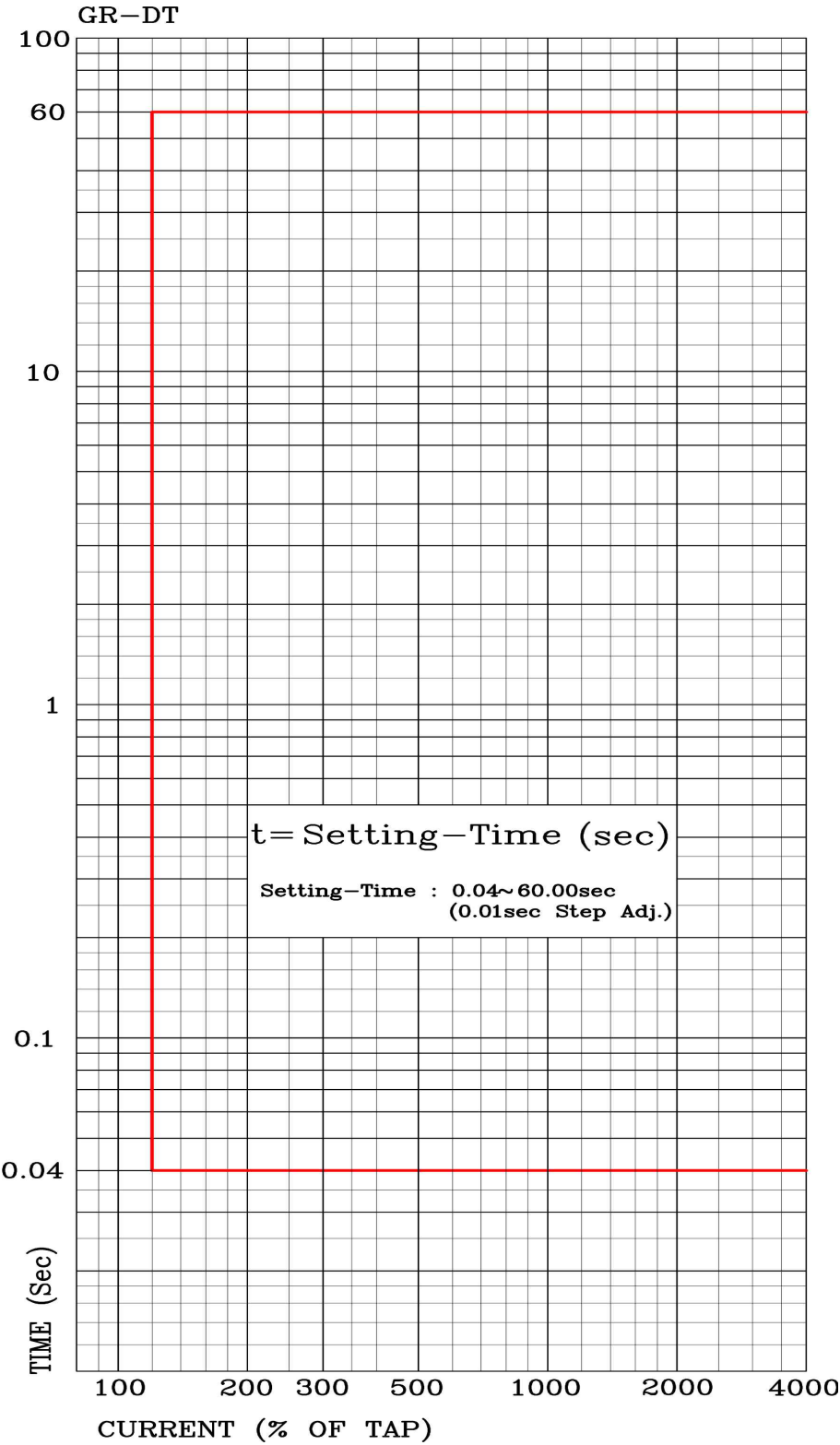
【부도 16】 지락 요소 정한시 특성 곡선
