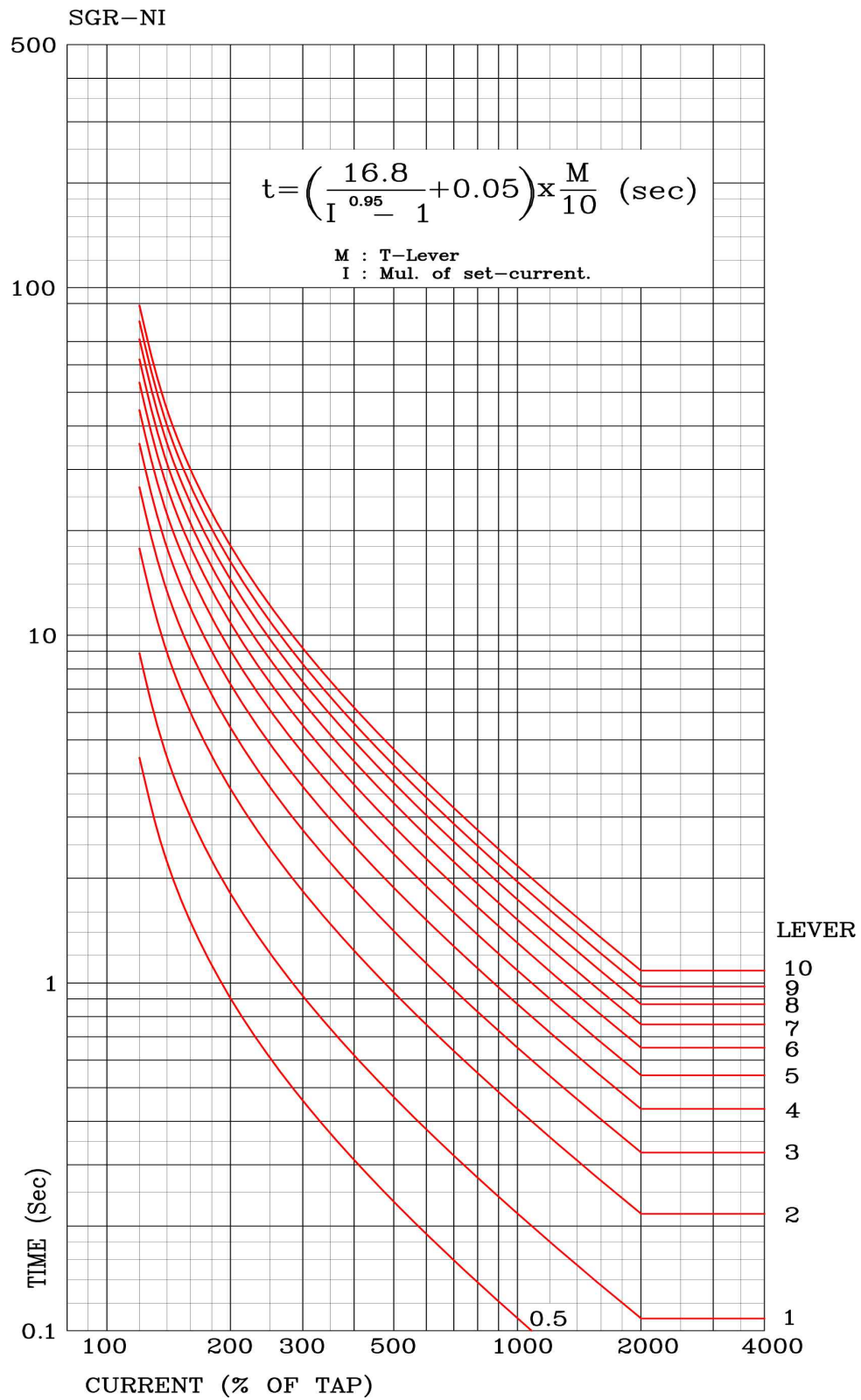
【부도 13】 선택 지락 / 지락 요소 반한시 특성 곡선
