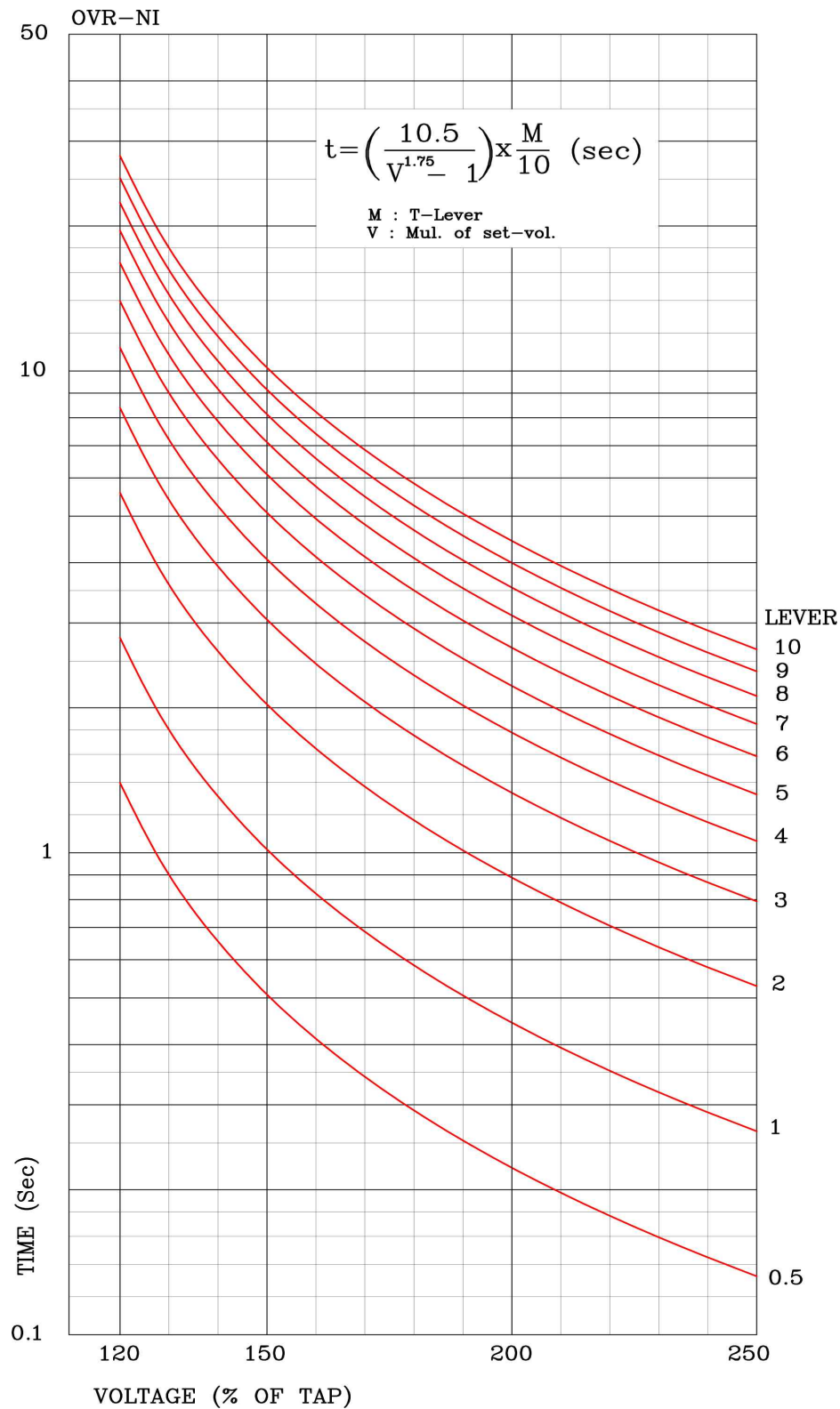
【부도 17】 과전압 요소 반한시 특성 곡선
