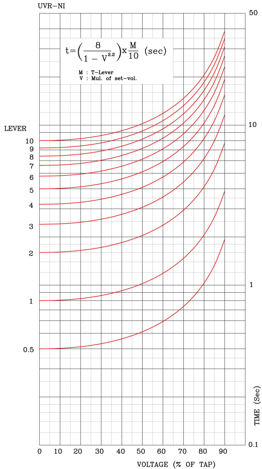
【부도 19】 저전압 요소 반환시 특성 곡선
