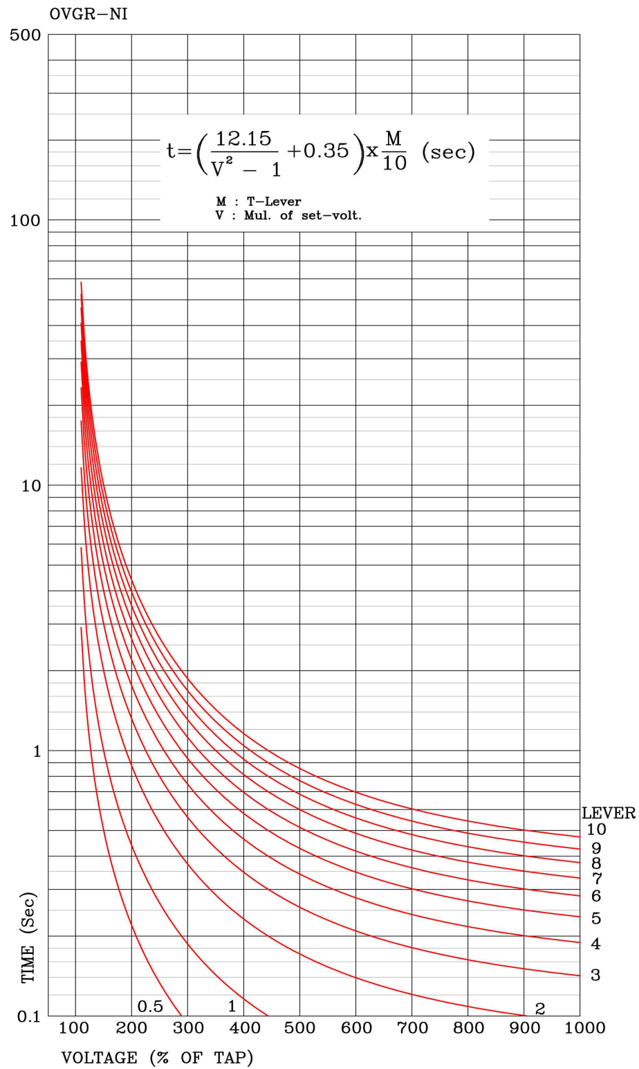
【부도 21】 지락 과전압 요소 반한시 특성 곡선
