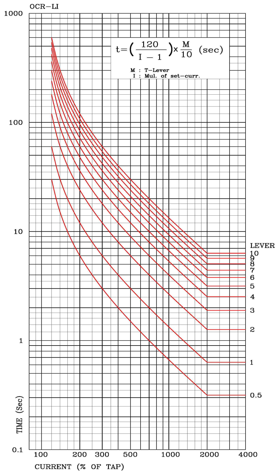
【부도 7】 과전류 요소 장반한시 특성 곡선
