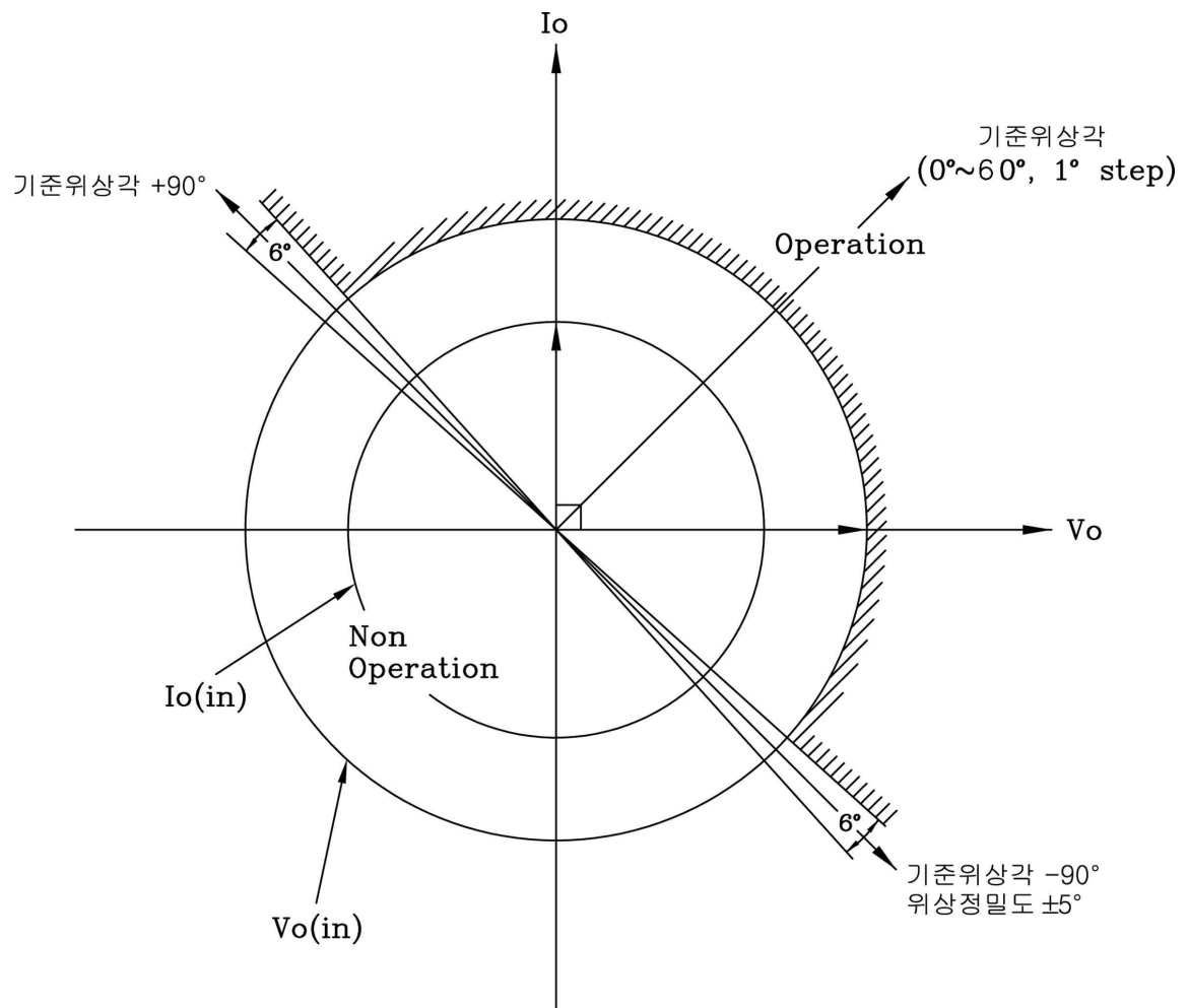
【부도 15】 선택 지락 요소 동작 특성 곡선
