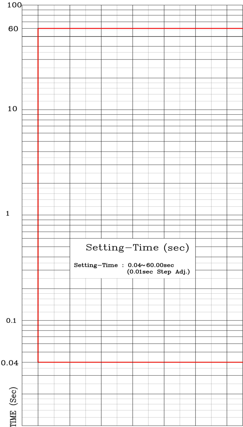
【부도 14】 선택 지락 요소 정한시 특성 곡선 SGR-DT
