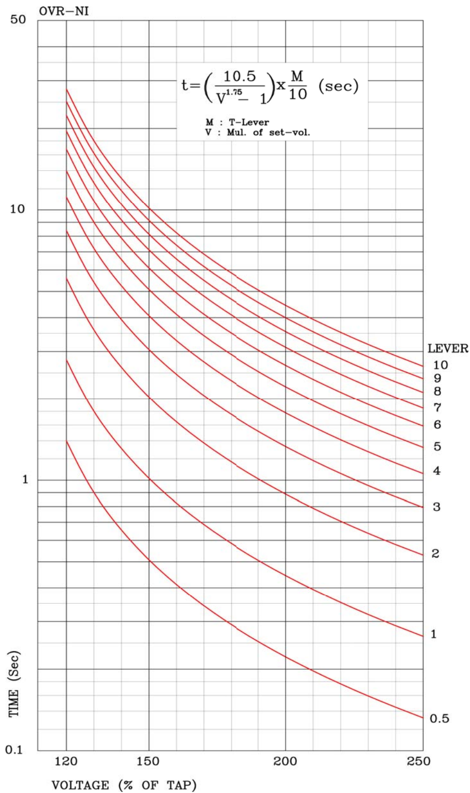
【부도 13】 과전압 요소 반한시 특성 곡선
