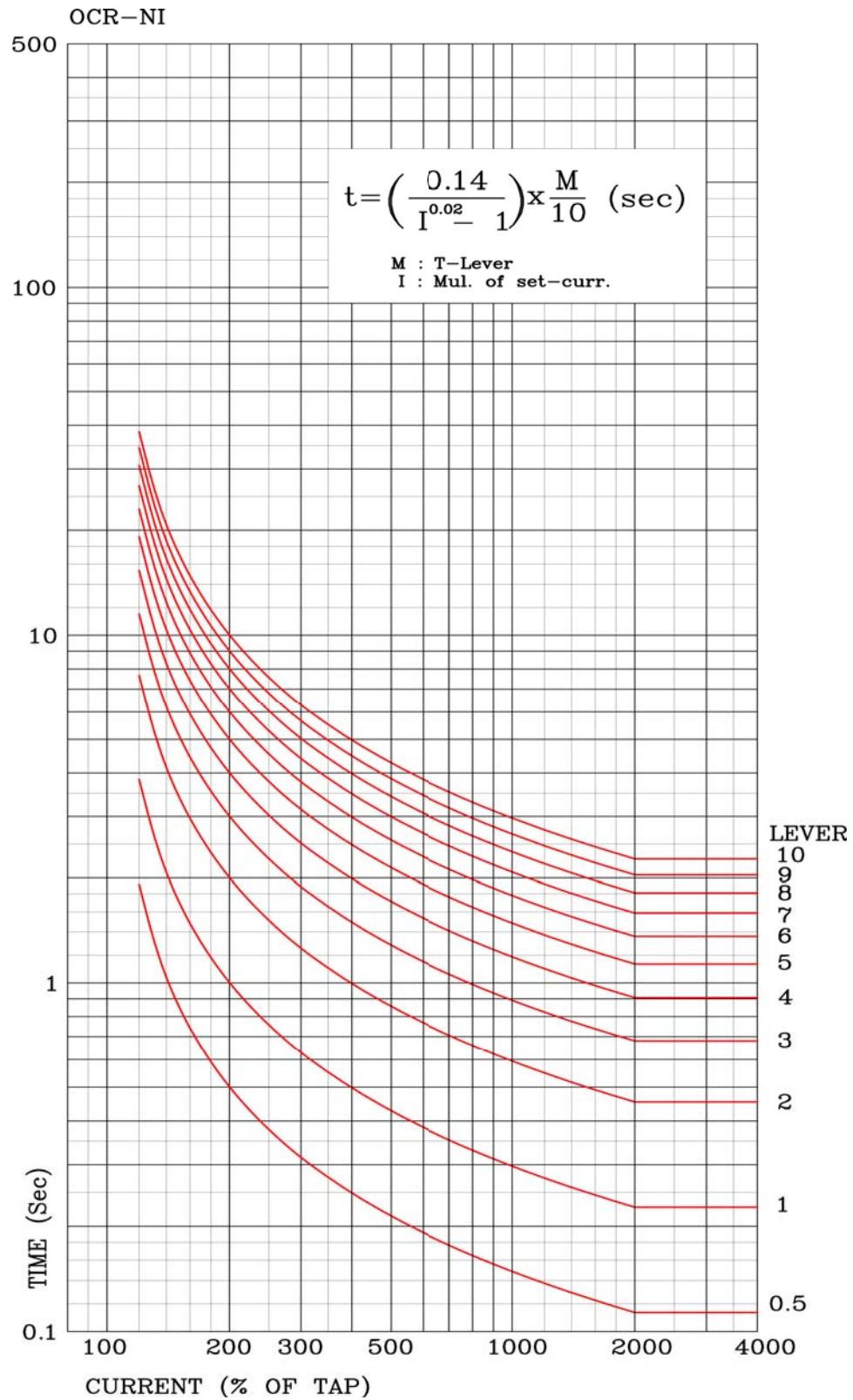
【부도 4】 과전류, 지락 과전류 요소 반한시 특성 곡선
