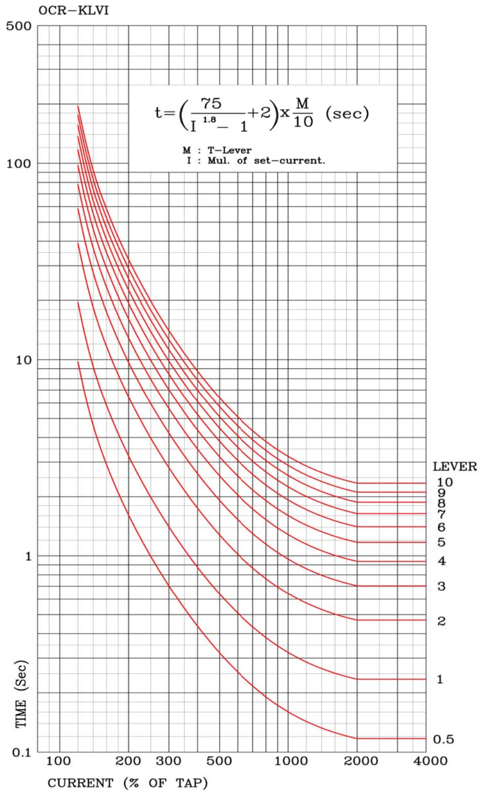
【부도 11】 과전류, 지락 과전류 요소 경보유도형 장강반한시 (KEPCO형) 특성 곡선
