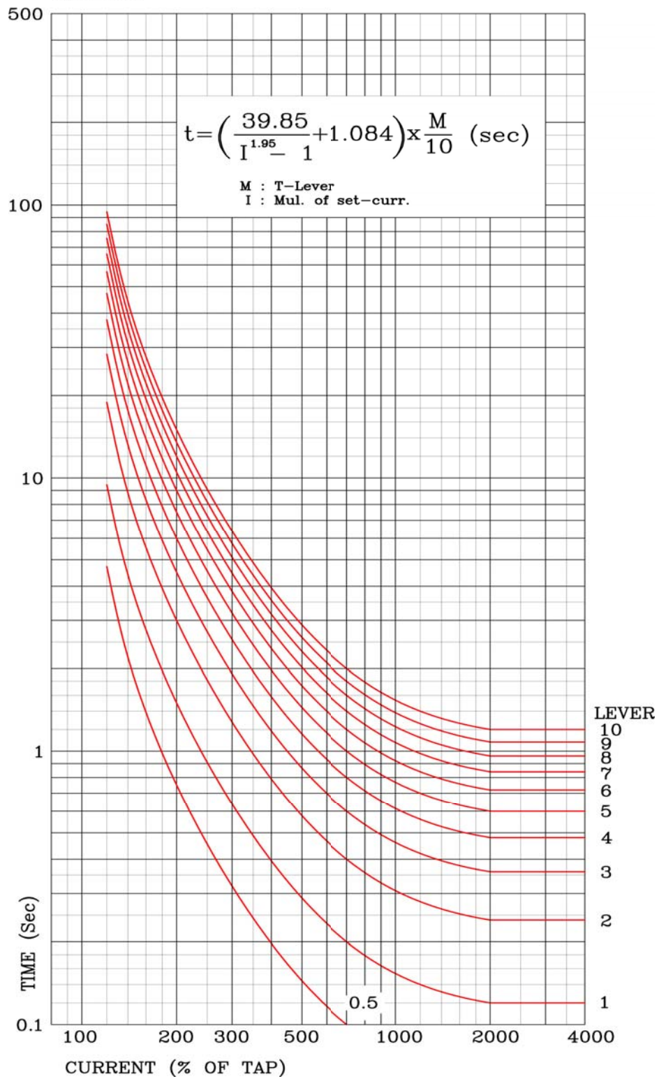
【부도 9】 과전류 요소, 지락 과전류 경보유도형 강제한시 (KEPCO형) 특성 곡선 OCR-KVI
