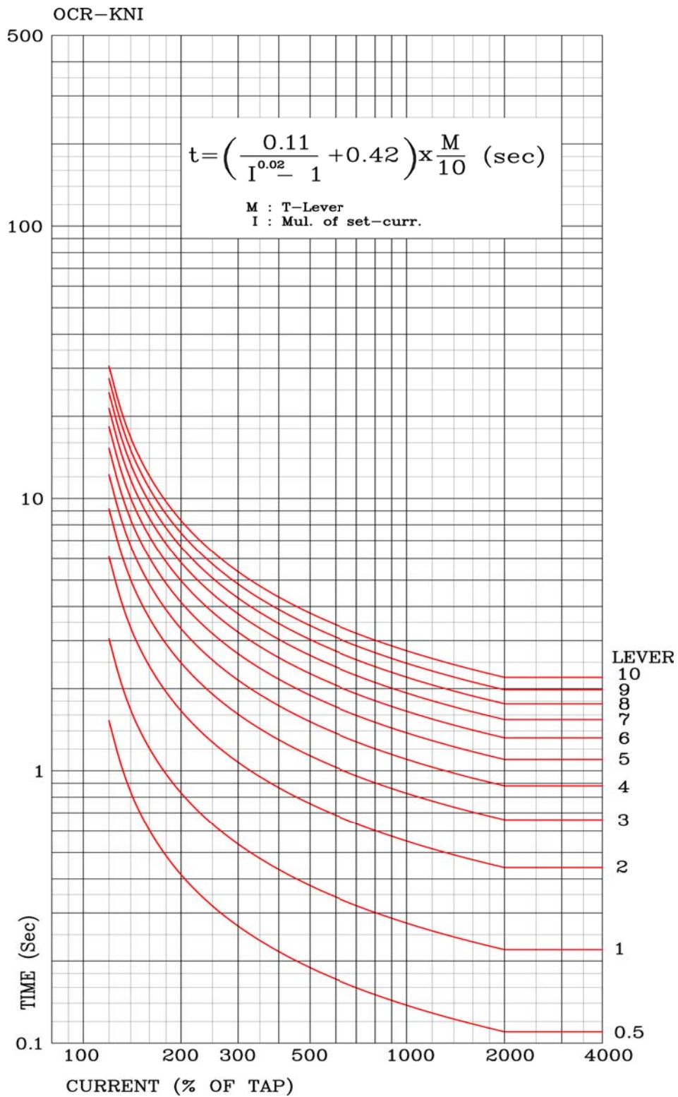
【부도 8】 과전류, 지락 과전류 요소 경보유도형 반한시 (KEPCO형) 특성 곡선
