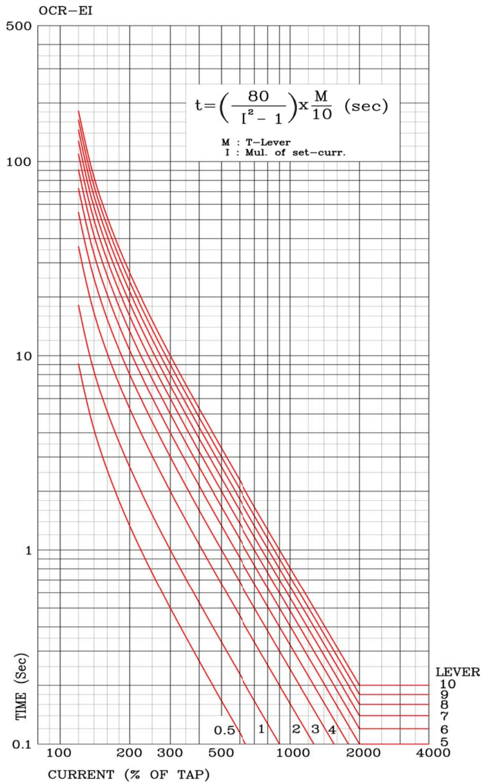
【부도 6】 과전류, 지락 과전류 요소 초반한시 특성 곡선
