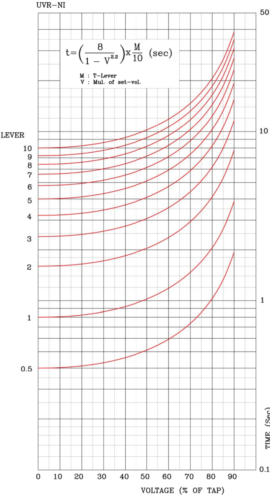
【부도 15】 저전압 요소 반환시 특성 곡선
