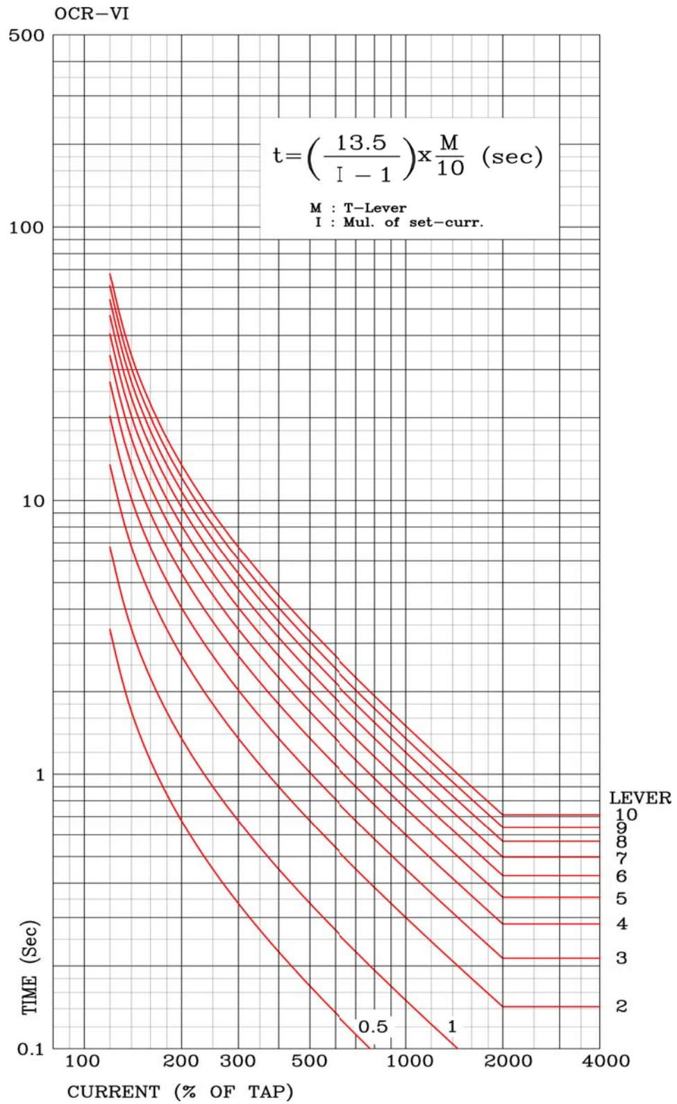
【부도 5】 과전류, 지락 과전류 요소 강제한시 특성 곡선
