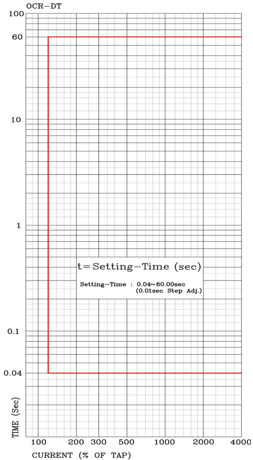
【부도 12】 과전류, 지락 과전류 요소 정한시 특성 곡선
