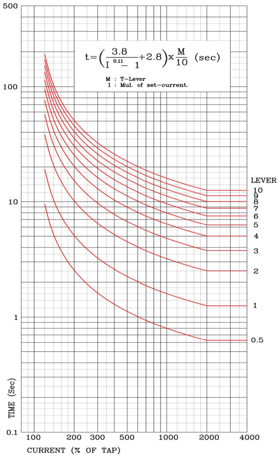
【부도 10】 과전류, 지락 과전류 요소 경보유도형 장반한시 (KEPCO형) 특성 곡선 OCR-KLNI
