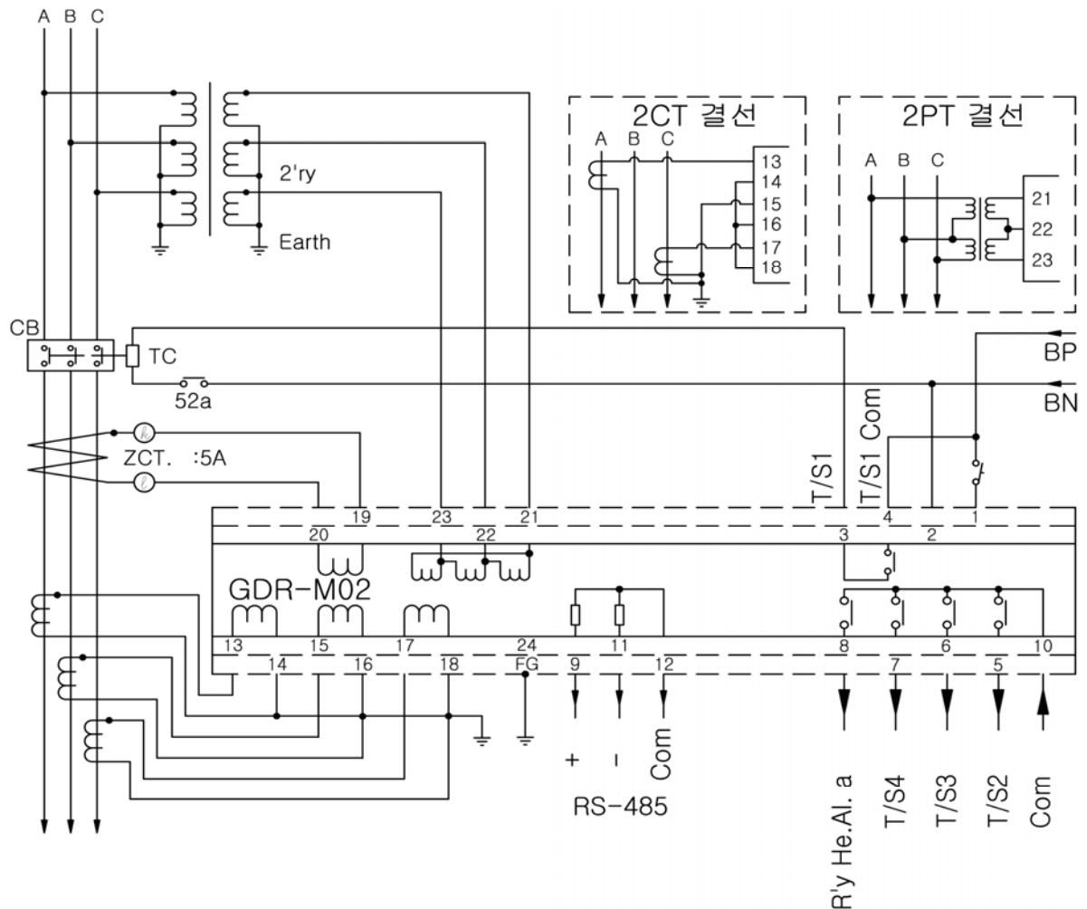
【부도 3】 외부 결선도
