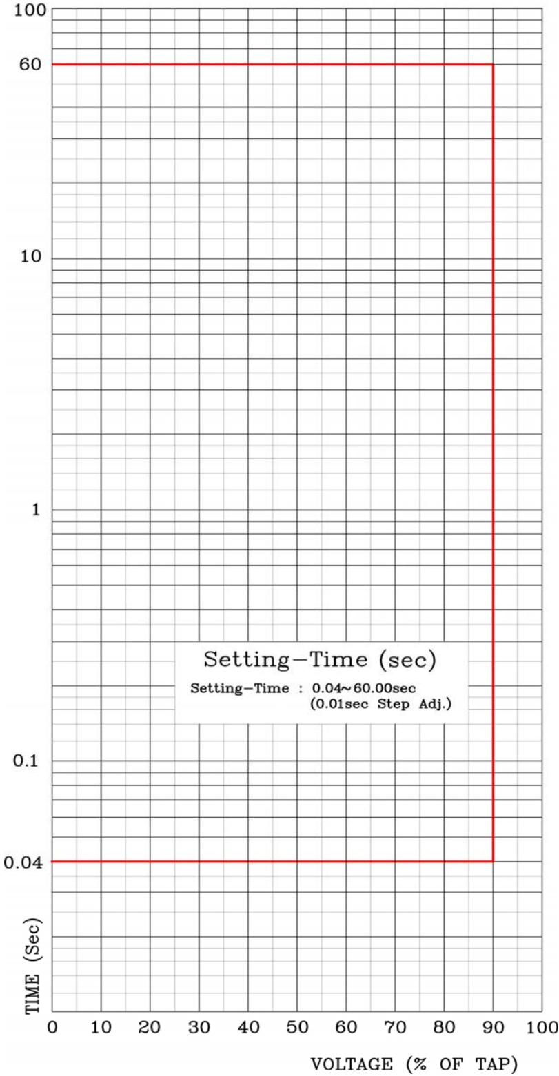
【부도 16】 저전압 요소 정한시 특성 곡선 UVR-DT
