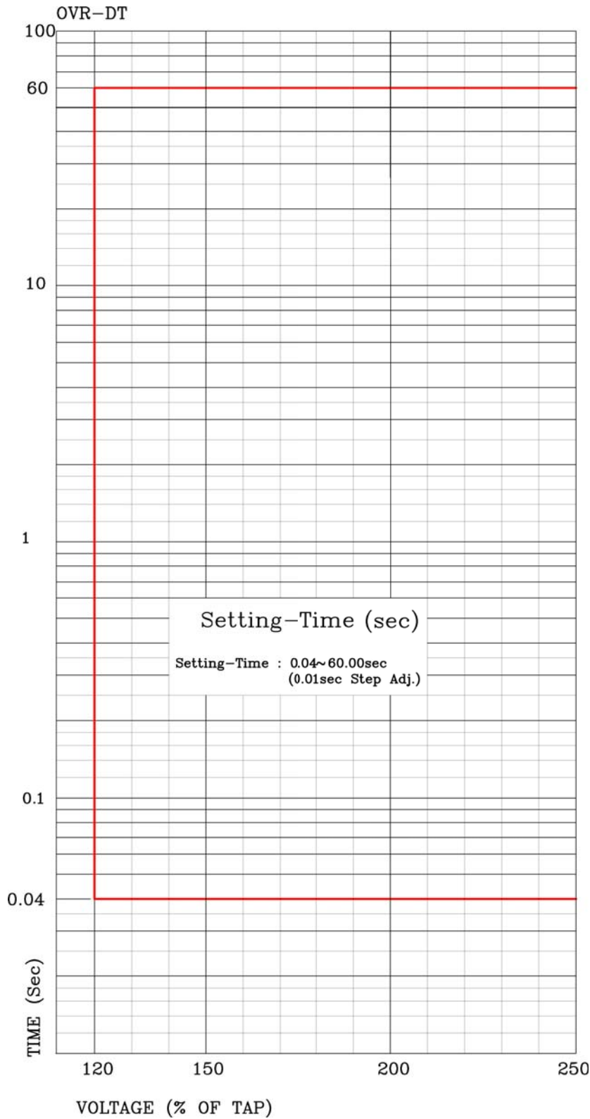
【부도 14】 과전압 요소 정한시 특성 곡선
