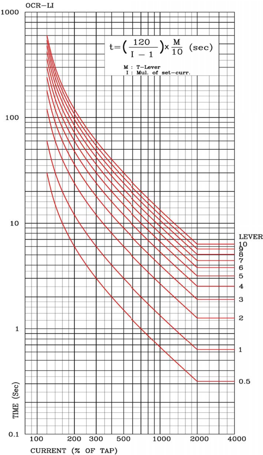
【부도 7】 과전류, 지락과전류 요소 장반한시 특성 곡선
