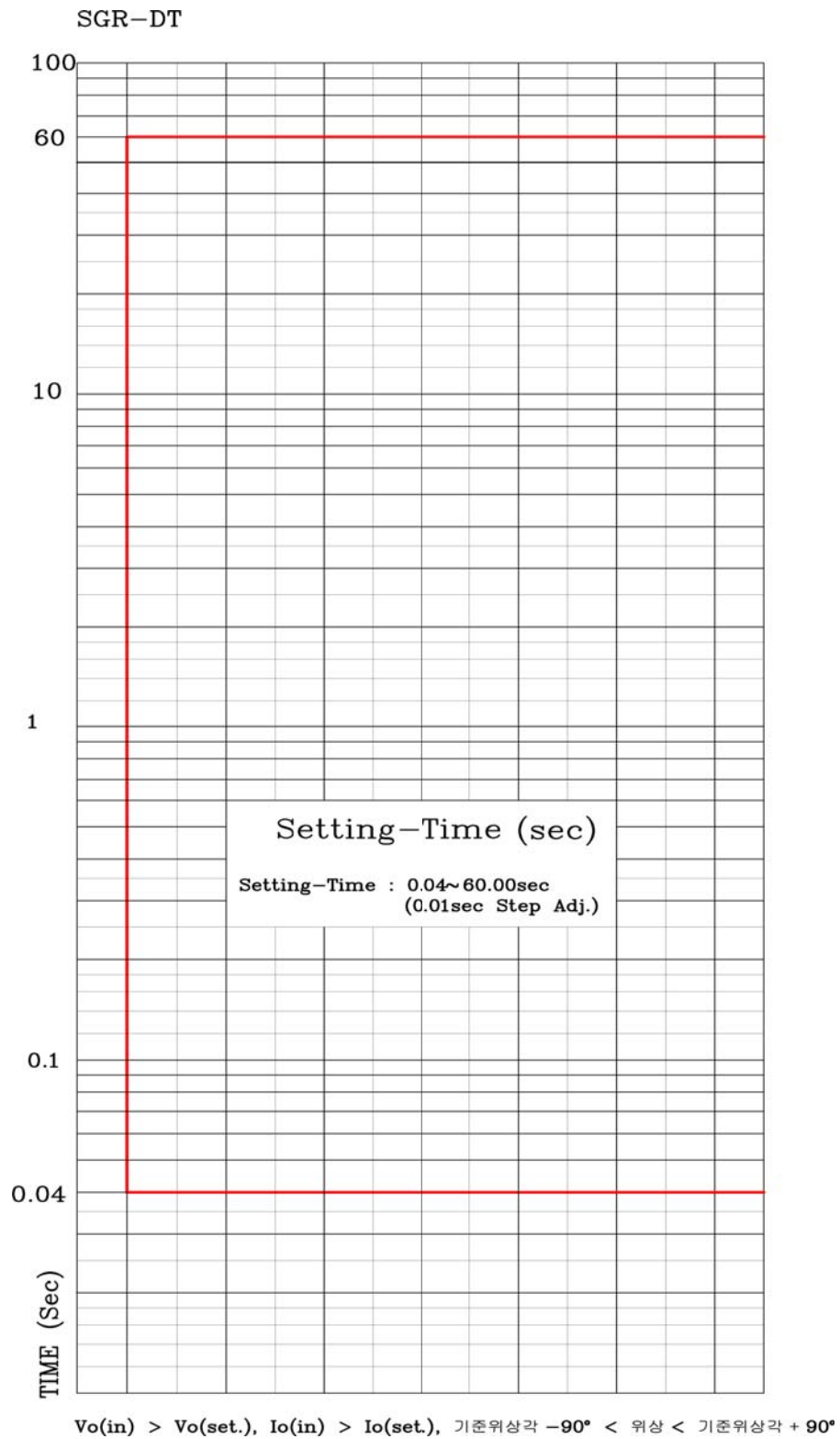
【부도 5】 정한시 특성 곡선
