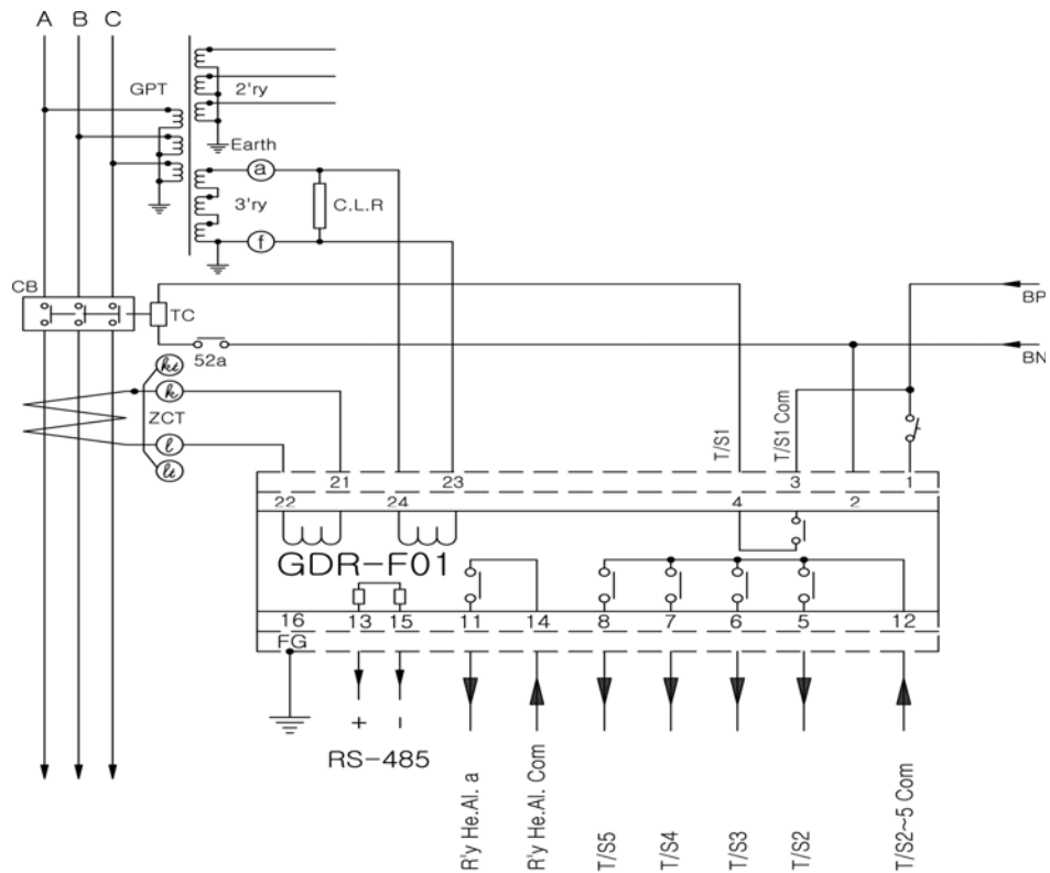
【부도 3】 외부 결선도
