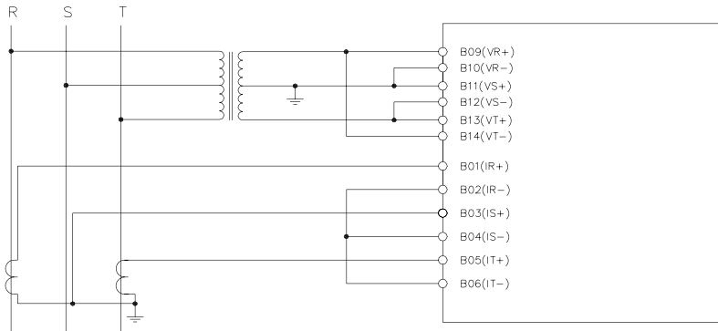
(3) 3P 3W : 2CT, 2PT
