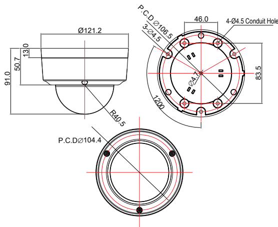
▲ FW7502-FTF 2MP 고정초점 반달프루프 돔카메라
