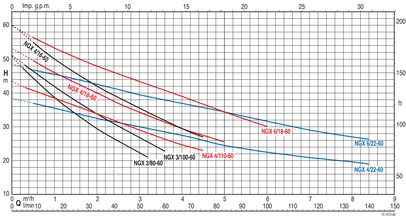
Coverage chart - Campo de aplicaciones n ≈ 3450 1/min
