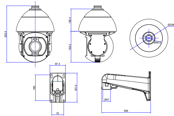
FW8707-FNR 2메가픽셀 레이저, IR 스피드돔 카메라
