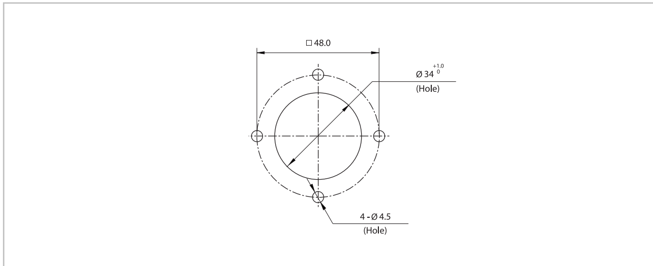
패널 가공 치수 | Panel cut-out dimension |
