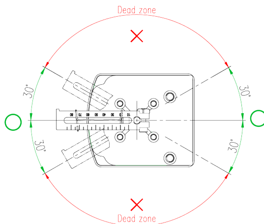
<리니어형 유효각도>
