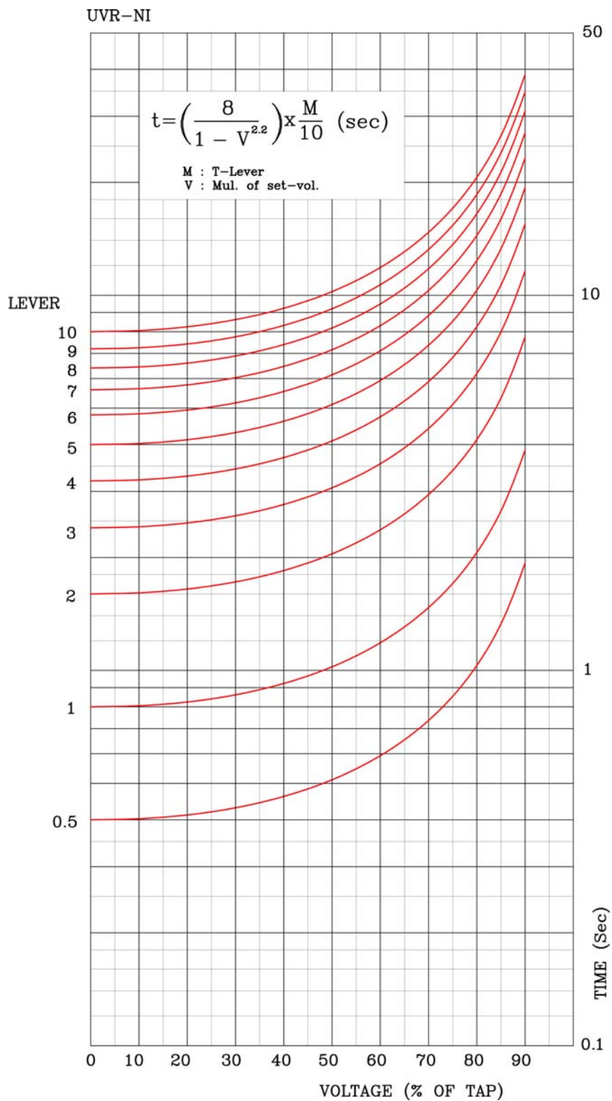
【부도 6】 저전압 요소 반한시 특성 곡선
