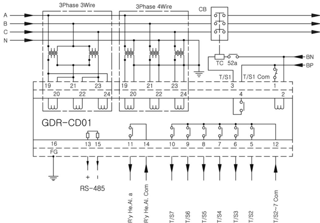
【부도 3】 외부 결선도
