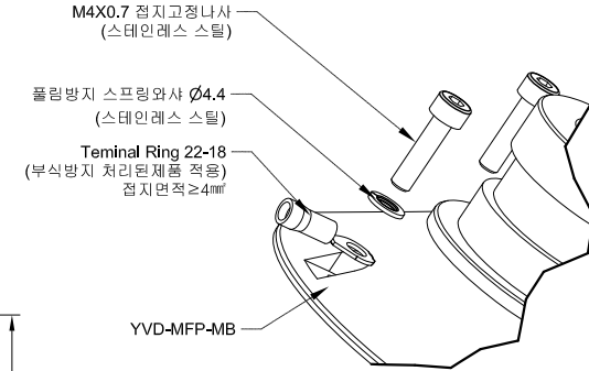
상세도 B
