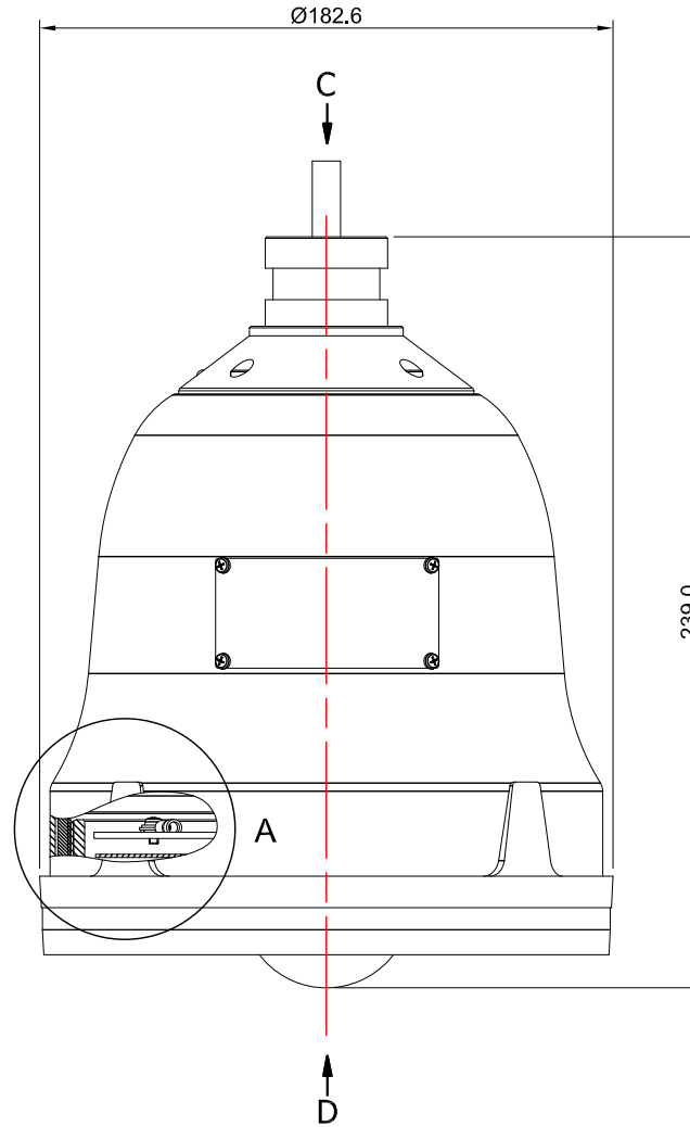
전면도
