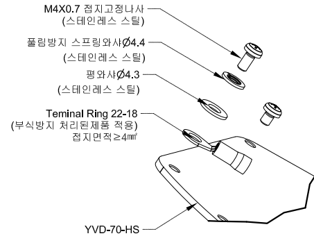
상세도 A
