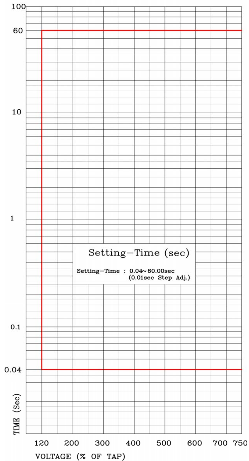
【부도 14】 지락 과전압 요소 정한시 특성 곡선 OVGR-DT
