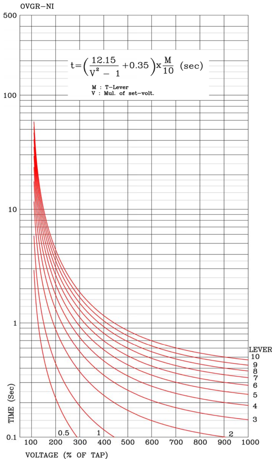
【부도 13】 지락 과전압 요소 반한시 특성 곡선
