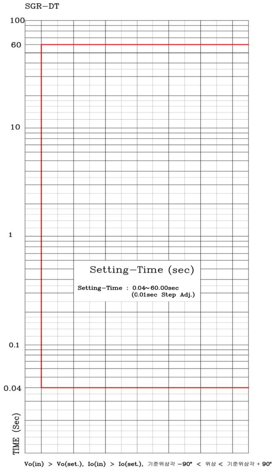
【부도 16】 선택 지락 요소 정한시 특성 곡선
