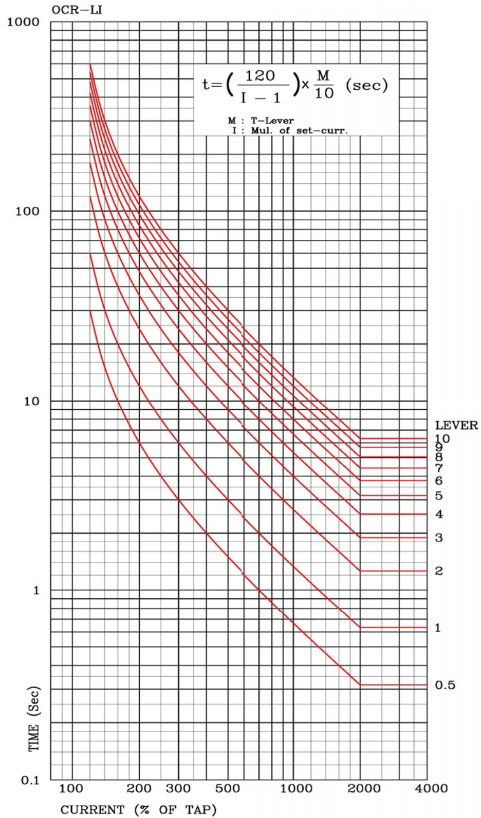
【부도 7】 과전류 요소 장반한시 특성 곡선
