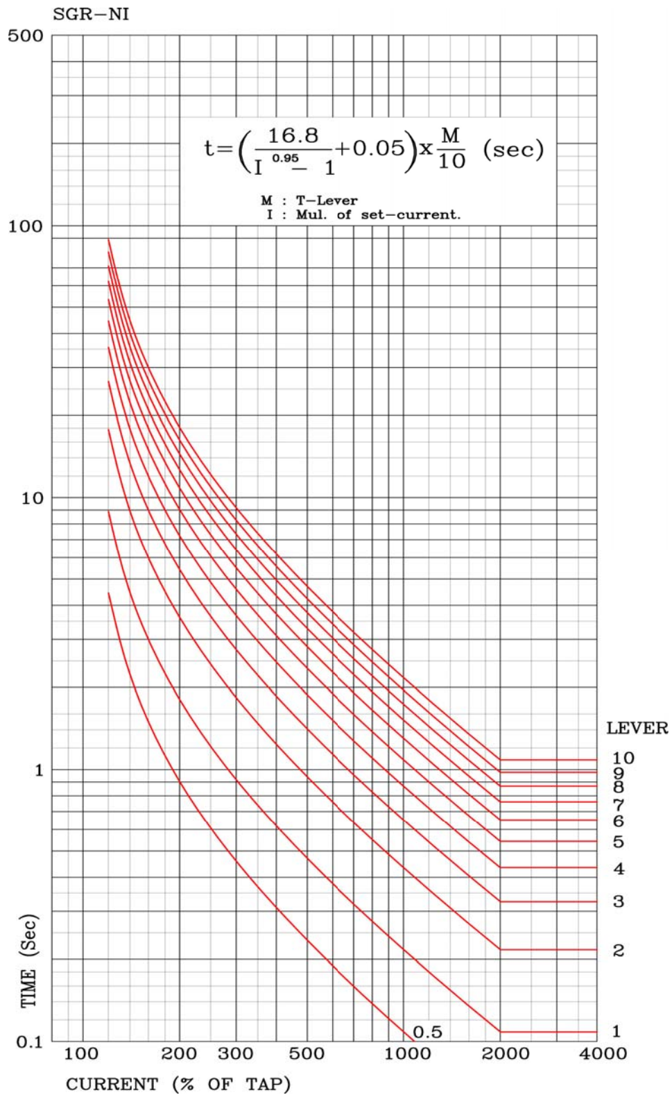
【부도 15】 선택 지락 요소 반한시 특성 곡선
