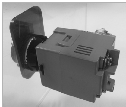
(3) 접점부를 홀다부에 밀어 끼운다 (Push the contact part into the holder part)
