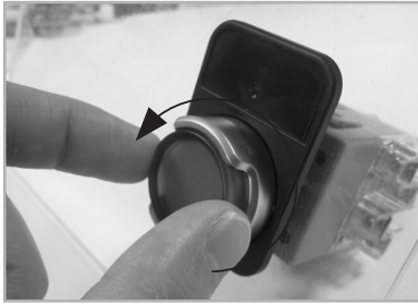
(1) 전면캡 반시계 방향으로 회전하여 캡을 제거 (Remove the CAP to turn counterclockwise)
