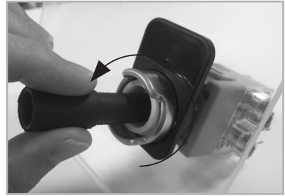
(3) LED 공구를 누른 후 반시계 방향으로 회전시켜 LED 램프 분리 (Remove the LED lamp to press the LED too and turn it counterclockwise)
