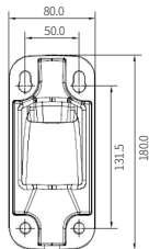
벽부형 브라켓
