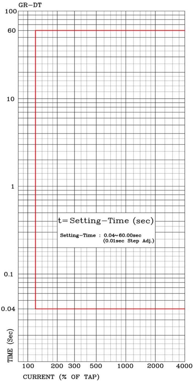
【부도 5】 정한시 특성 곡선
