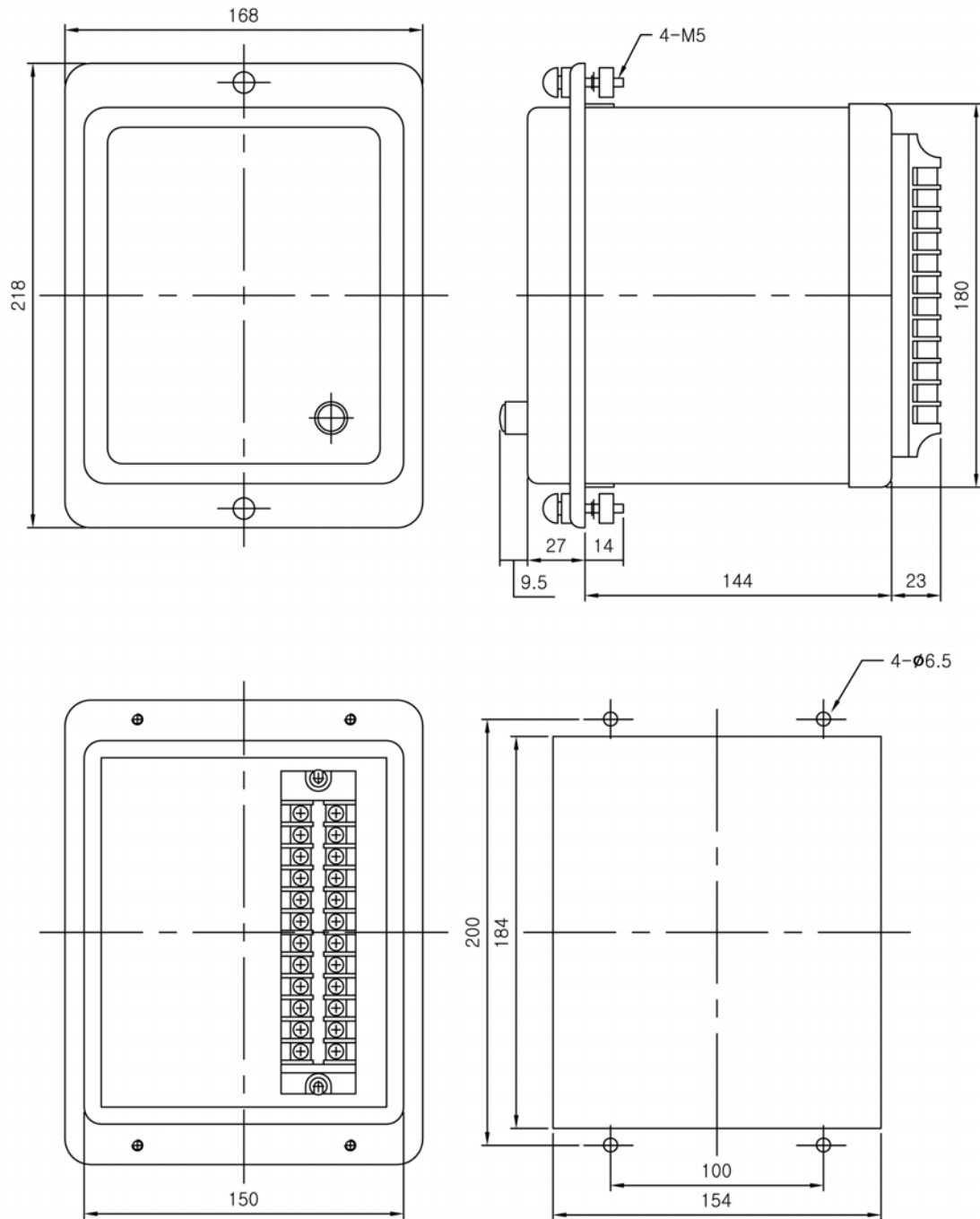
【부도 1】 계전기 외형 및 치수 ( Unit : mm )
