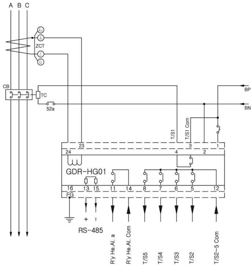
【부도 4】 외부 결선도
