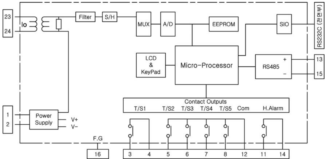
【부도 3】 내부 Block Diagram
