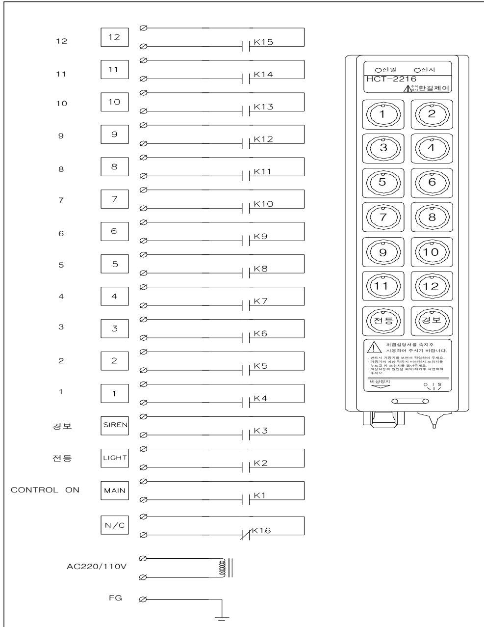
- 수신기 출력도
