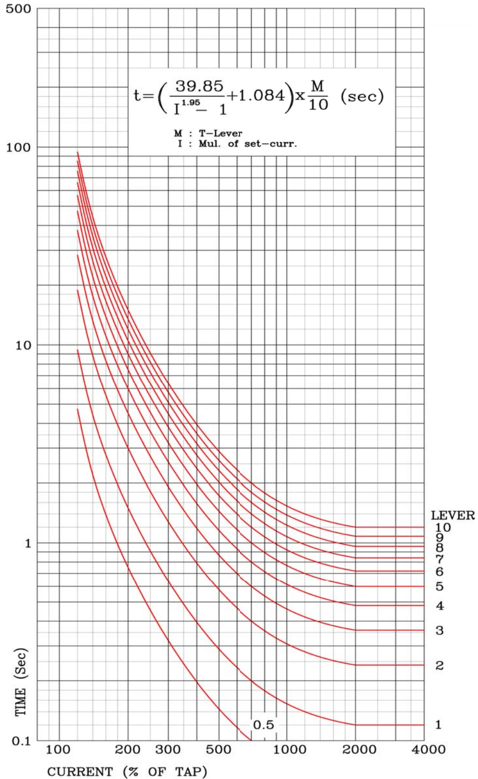
【부도 9】 과전류 요소 경보유도형 강반한시 (KEPCO형) 특성 곡선 OCR-KVI
