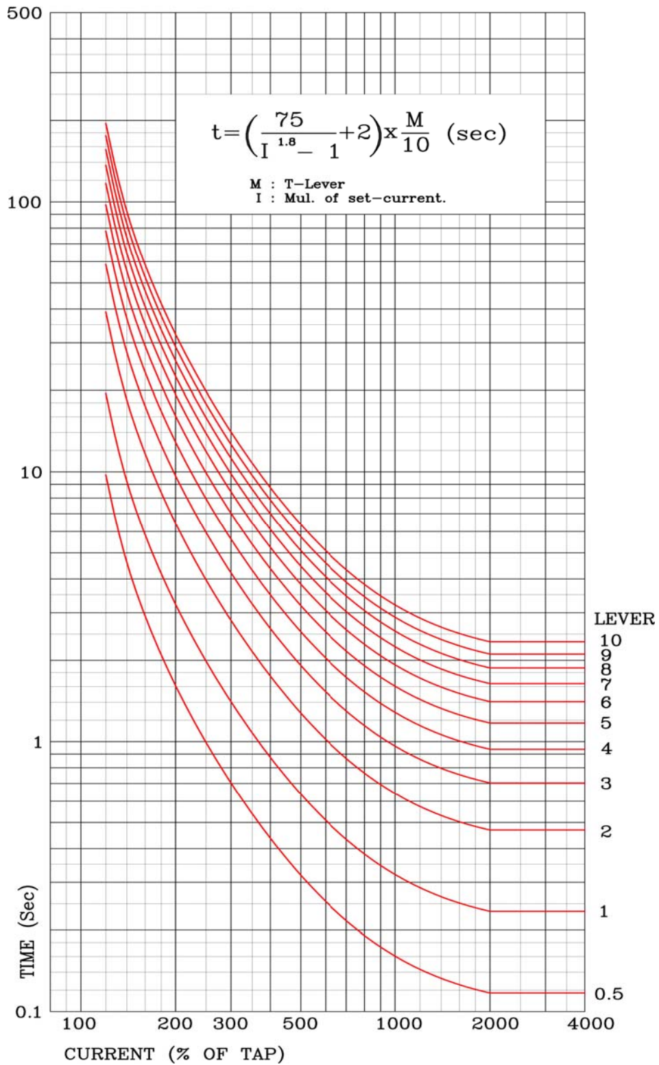
【부도 11】 과전류 요소 경보유도형 장강반한시 (KEPCO형) 특성 곡선 OCR-KLVI
