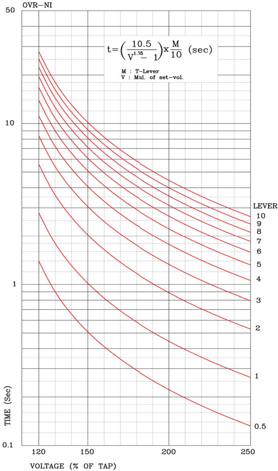
【부도 13】 과전압 요소 반환시 특성 곡선
