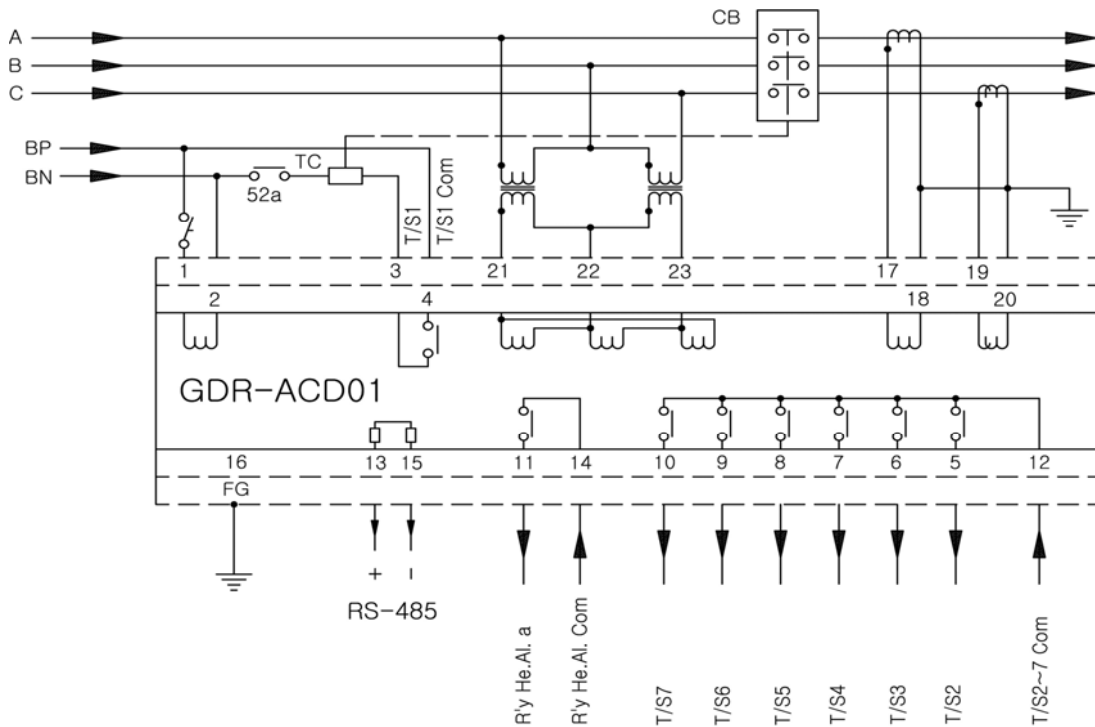
【부도 3】 외부 결선도
