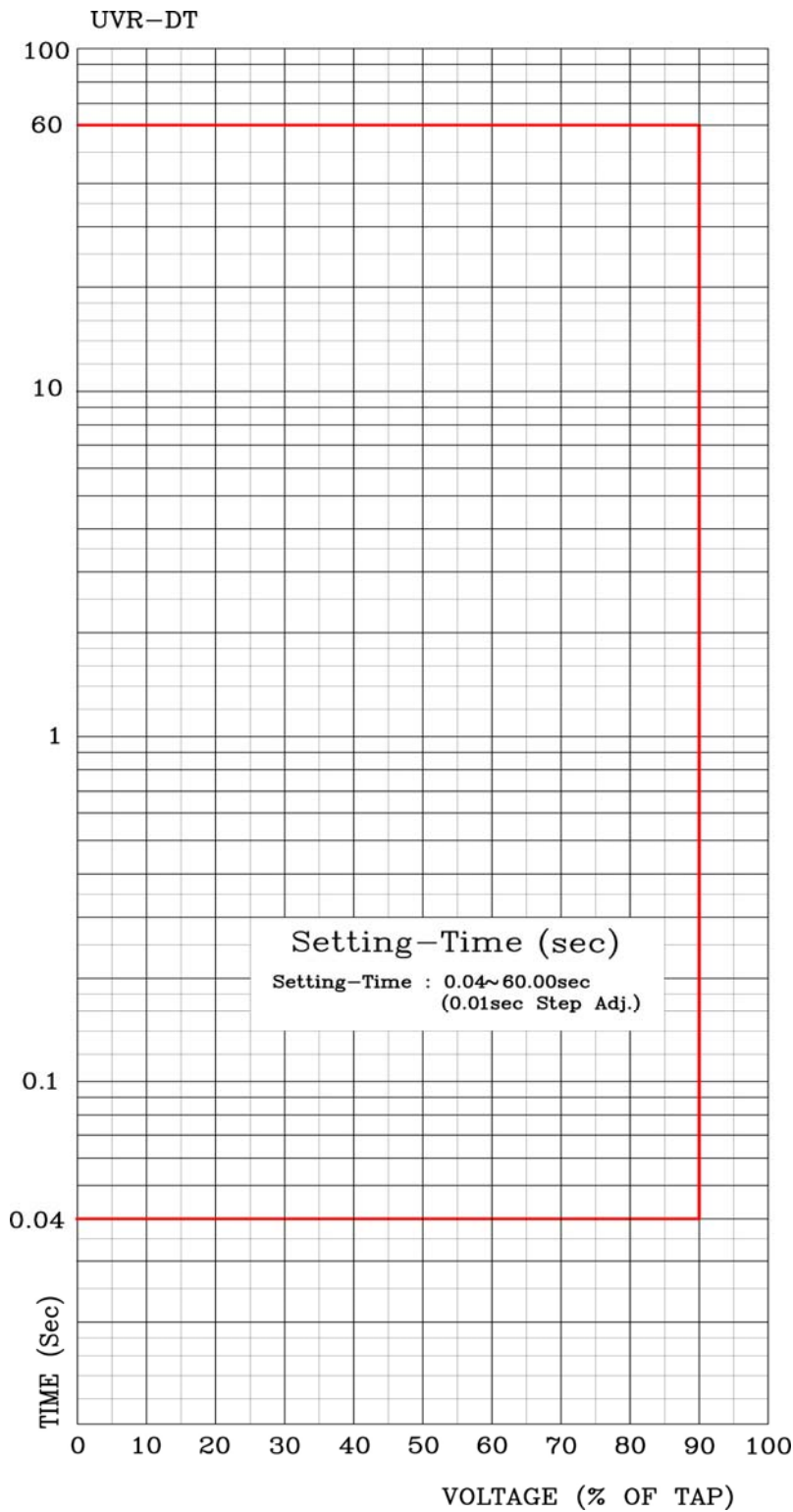
【부도 16】 저전압 요소 정한시 특성 곡선
