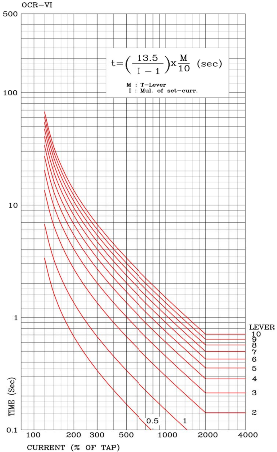
【부도 5】 과전류 요소 강반한시 특성 곡선
