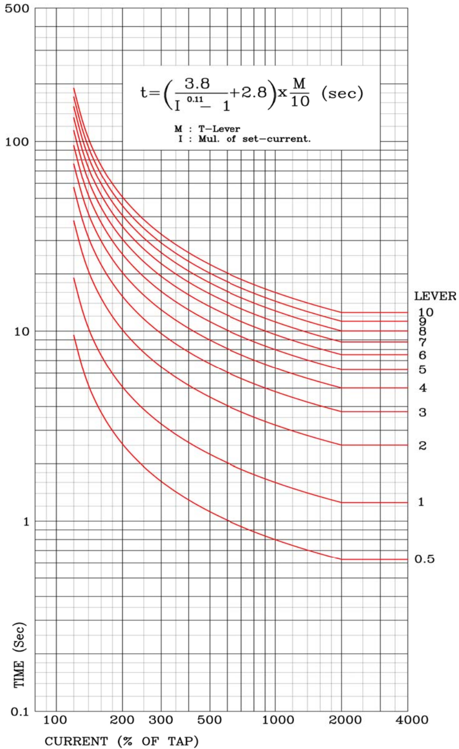
【부도 10】 과전류 요소 경보유도형 장반한시 (KEPCO형) 특성 곡선 OCR-KLNI
