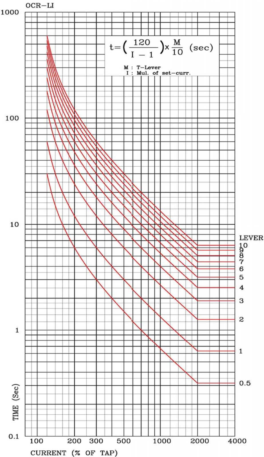
【부도 7】 과전류 요소 장반한시 특성 곡선
