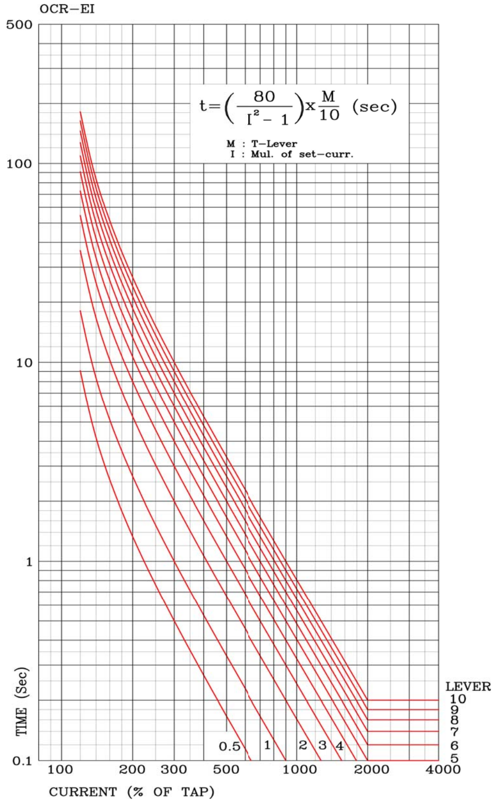
【부도 6】 과전류 요소 초반한시 특성 곡선
