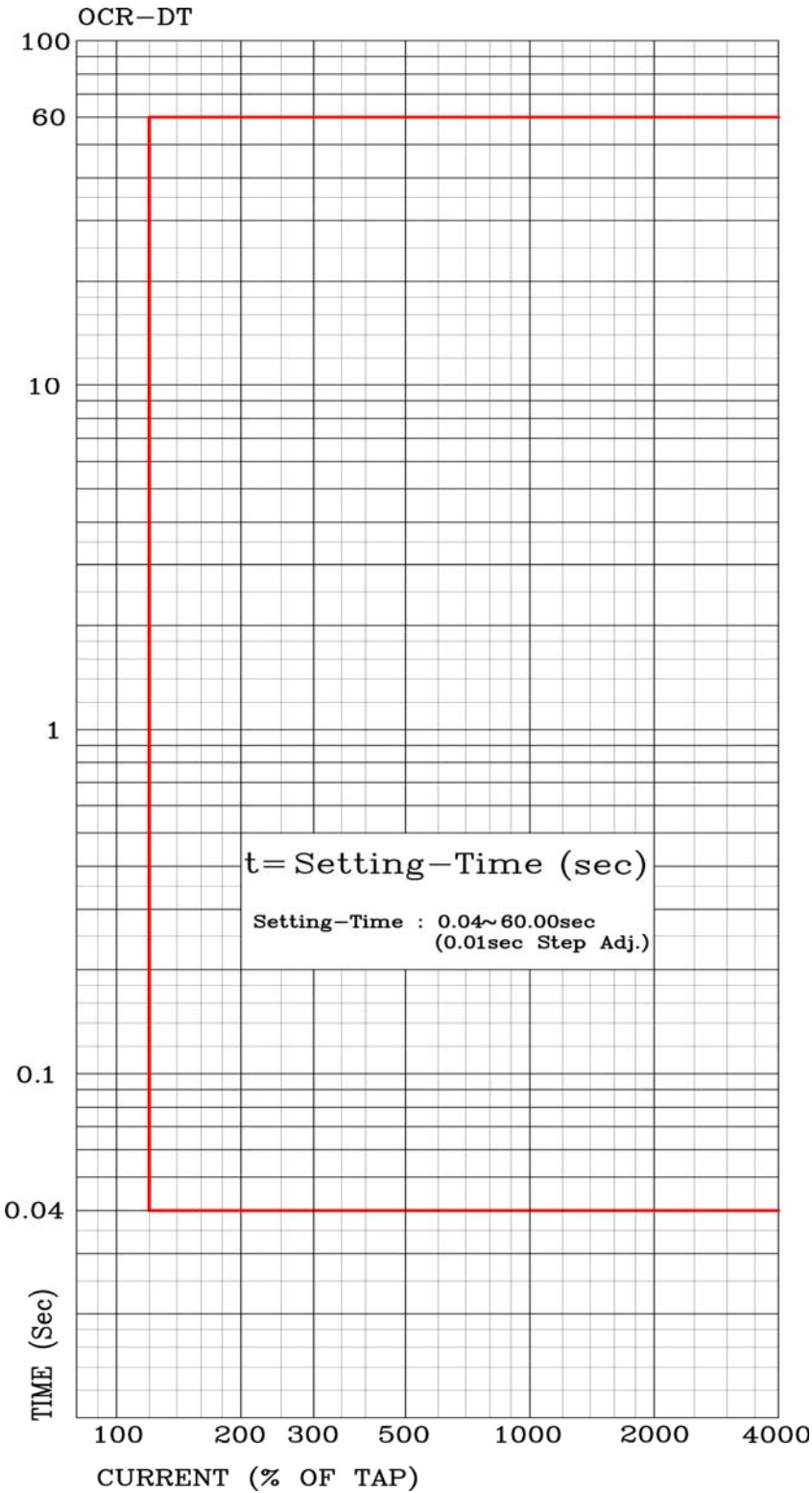
【부도 12】 과전류 요소 정한시 특성 곡선
