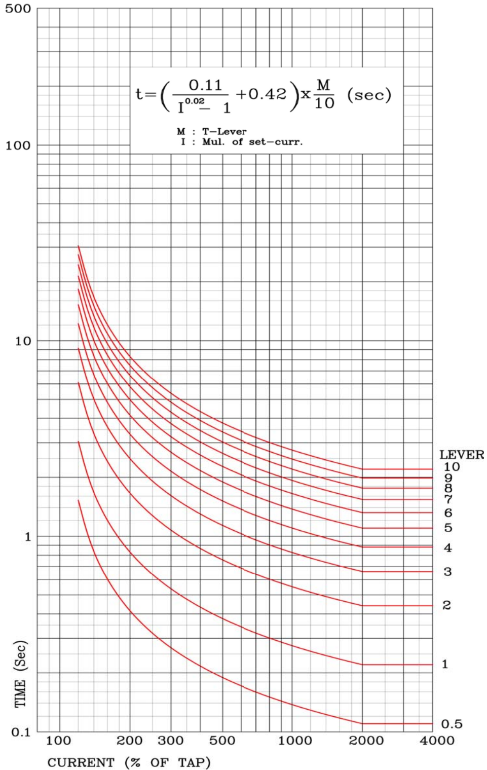
【부도 8】 과전류 요소 경보유도형 반한시 (KEPCO형) 특성 곡선 OCR-KNI
