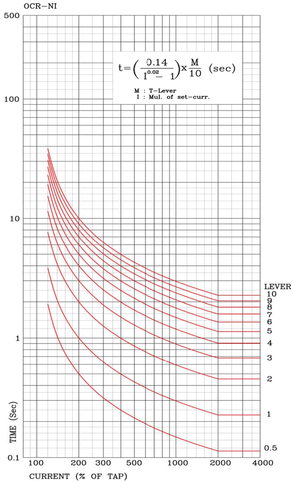
【부도 4】 과전류 요소 반한시 특성 곡선
