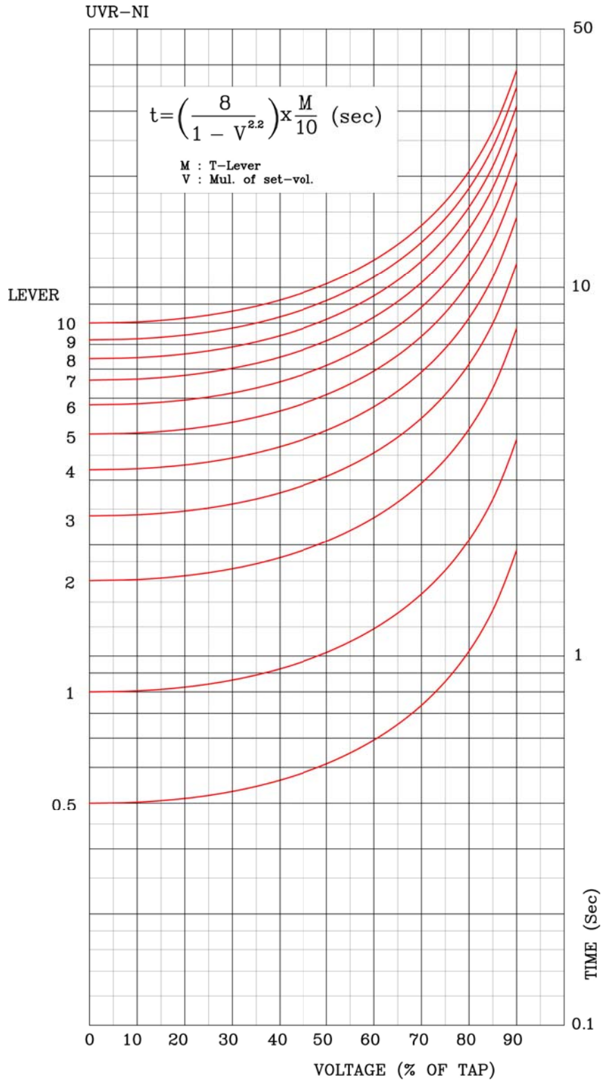
【부도 15】 저전압 요소 반한시 특성 곡선
