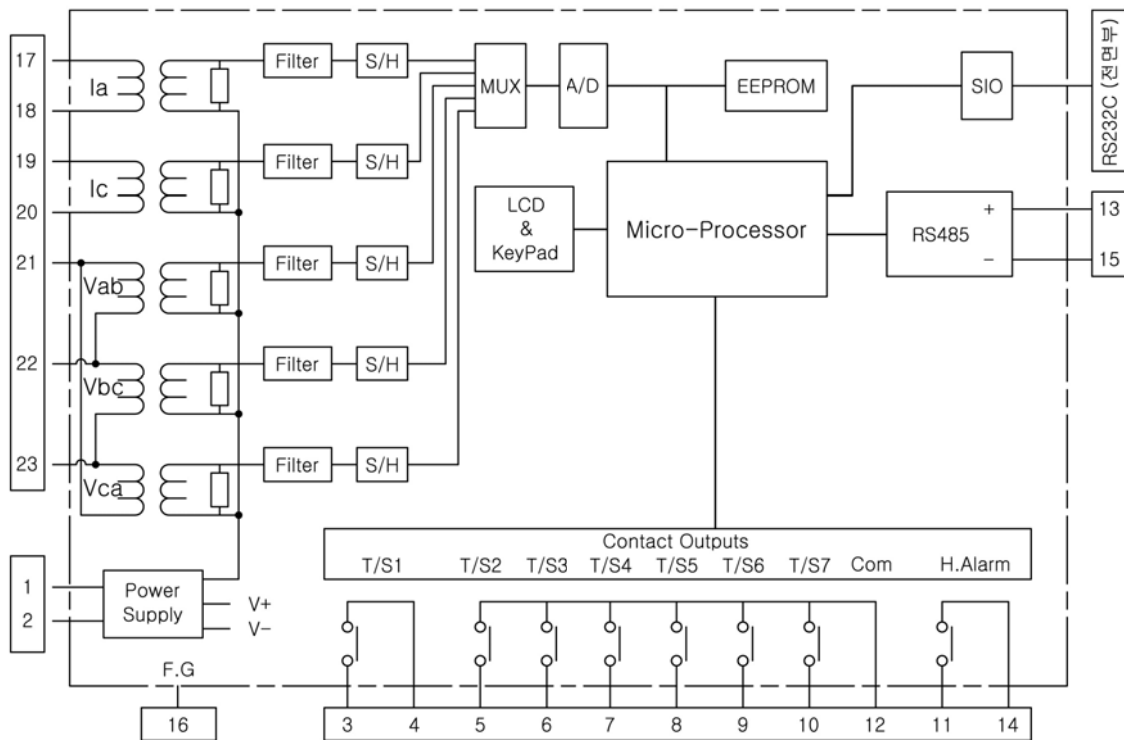
【부도 3】 외부 결선도
