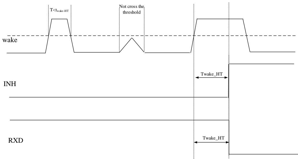
Figure 9-6. Local Wake Up – Rising Edge
