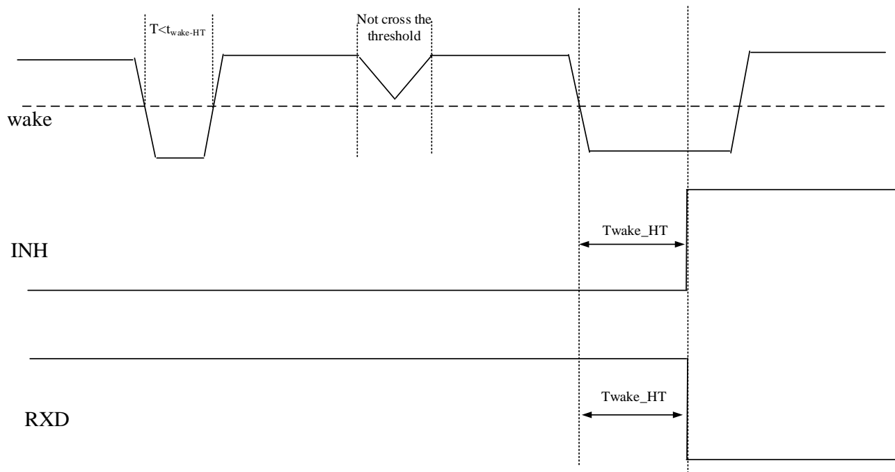
Figure 9-7. Local Wake Up – Falling Edge
