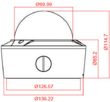
▲ FW7511-TVM 3MP Vandal proof Dome
