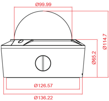
▲ FW7511-TVM 3MP 가변자동초점 반달프루프 돔 카메라
