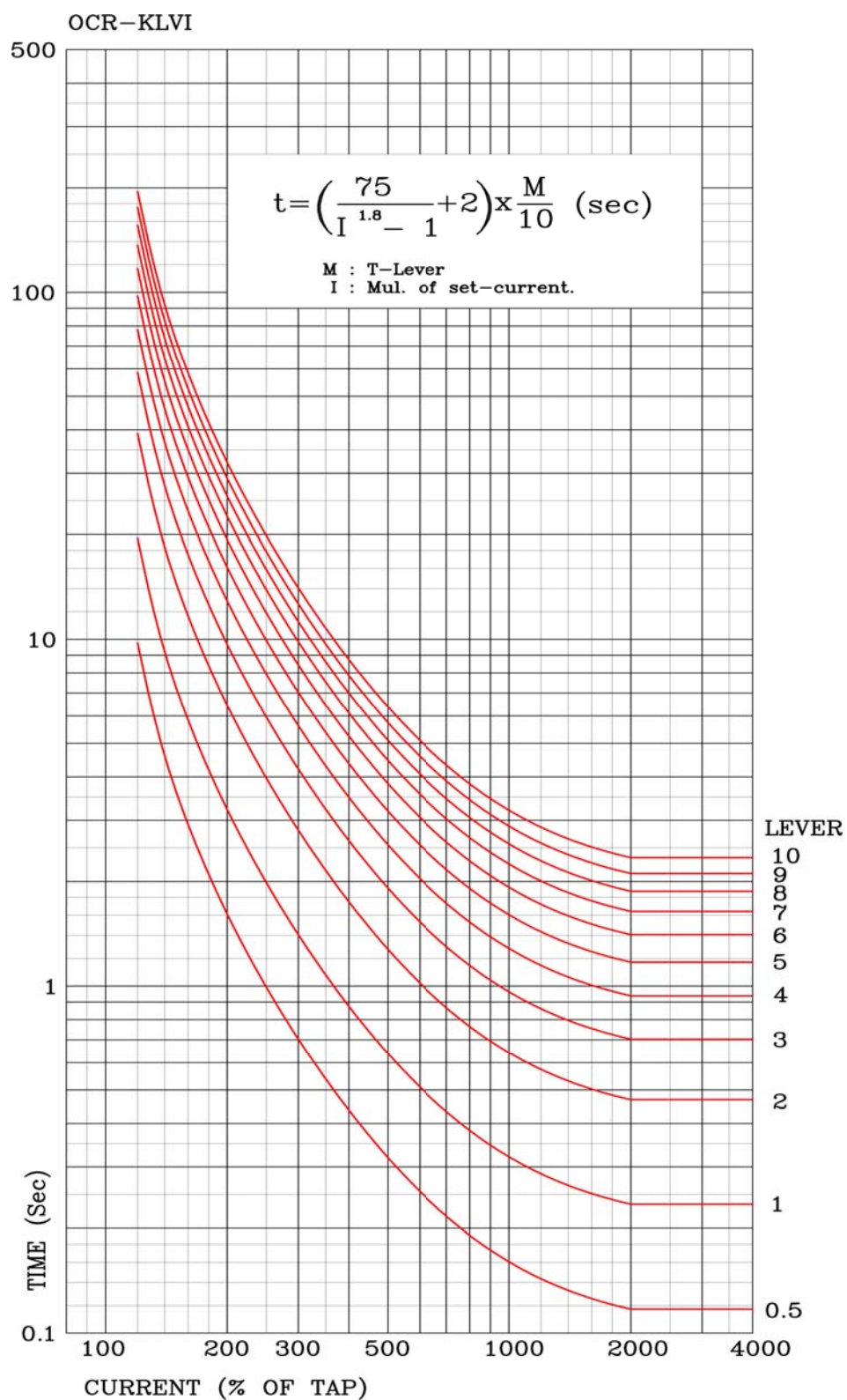
【부도 11】 경보유도형 장강반한시 (KEPCO형) 특성 곡선
