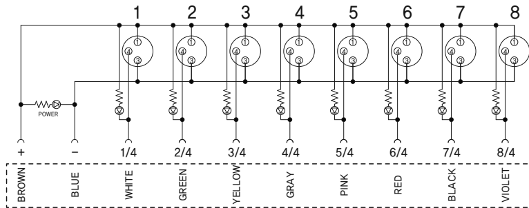
Cable Color
