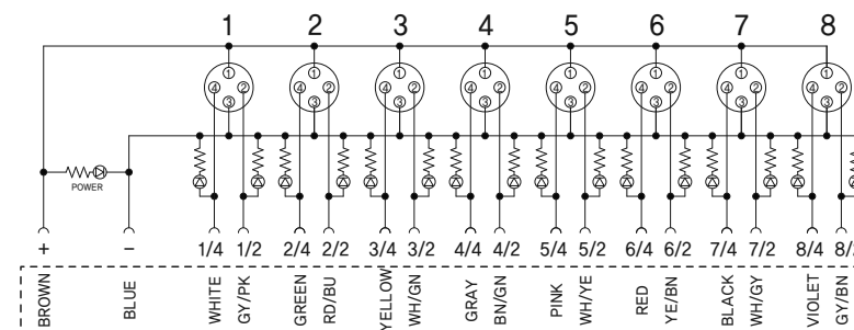
Cable Color
