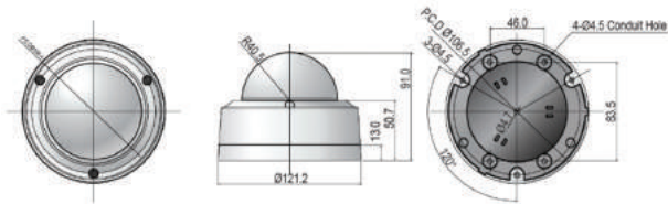
▲ FW7502-TVF 3MP Vandal proof Dome
