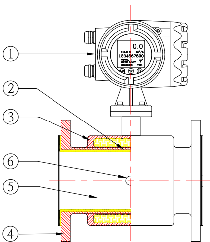
그림 1.2 구조도 (KTM-800)
