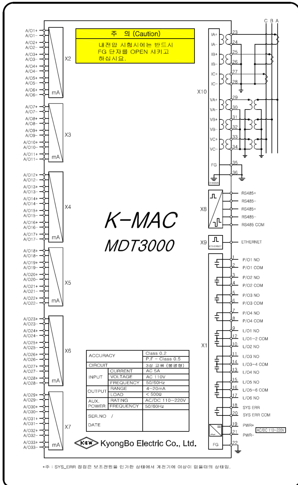
【부도 2】 K-MAC MDT3000 외부 결선도
