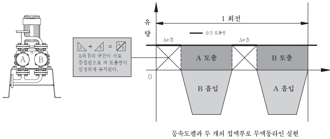
그림C 무맥동 정량펌프(DOUBLE HEAD)
