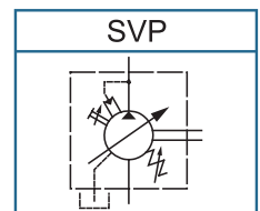
KS 유압기호도
