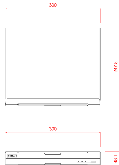
외관도 (단위 : mm)
