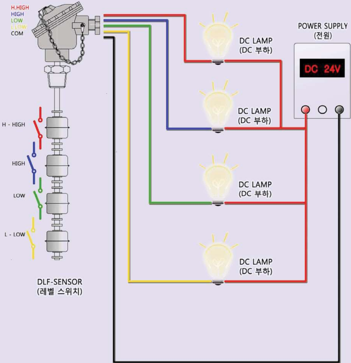
Wiring To a DC - POWER SUPPLY (DC 회로 연결시)
