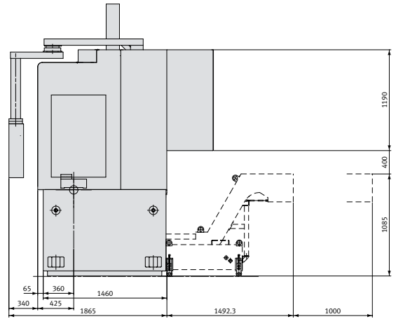
측면도
