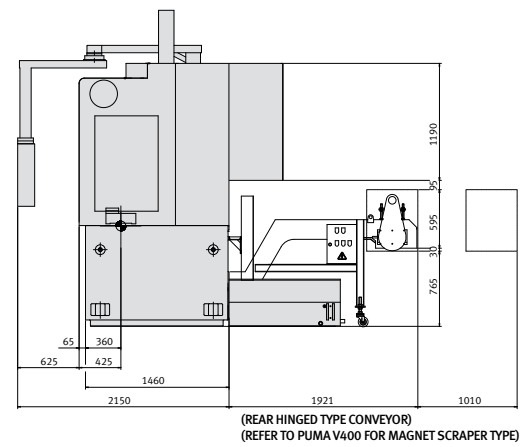
측면도
