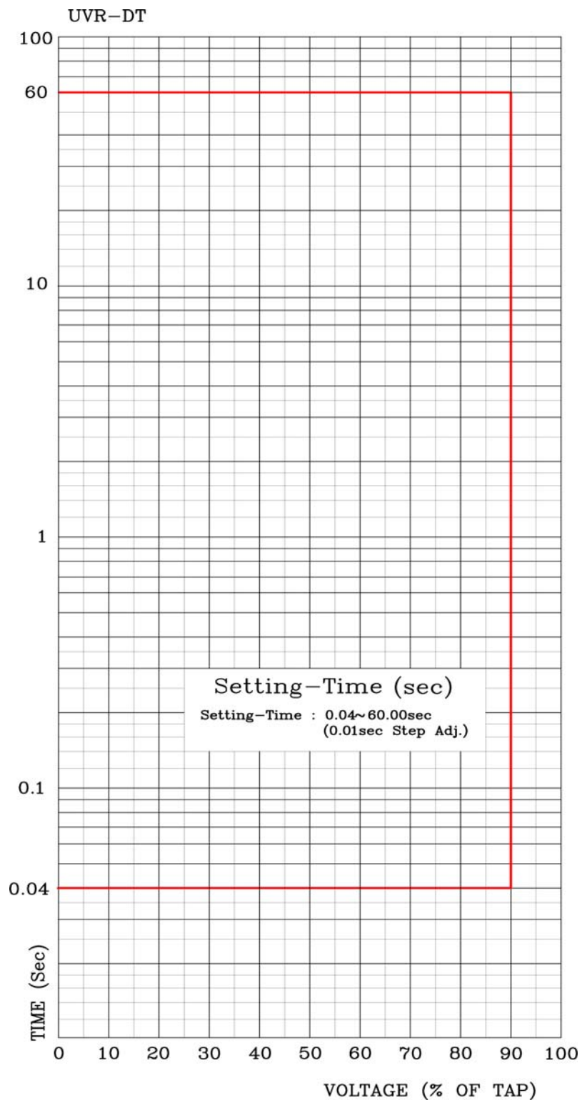
【부도 5】 정한시 특성 곡선
