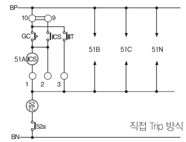
직접 Trip 방식
