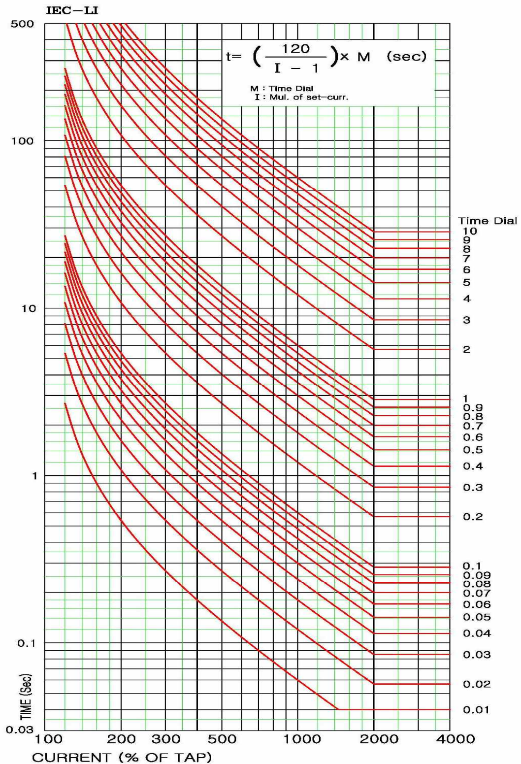
【부도 6】 과전류, 지락과전류, 역상과전류 IEC_LI 특성 곡선
