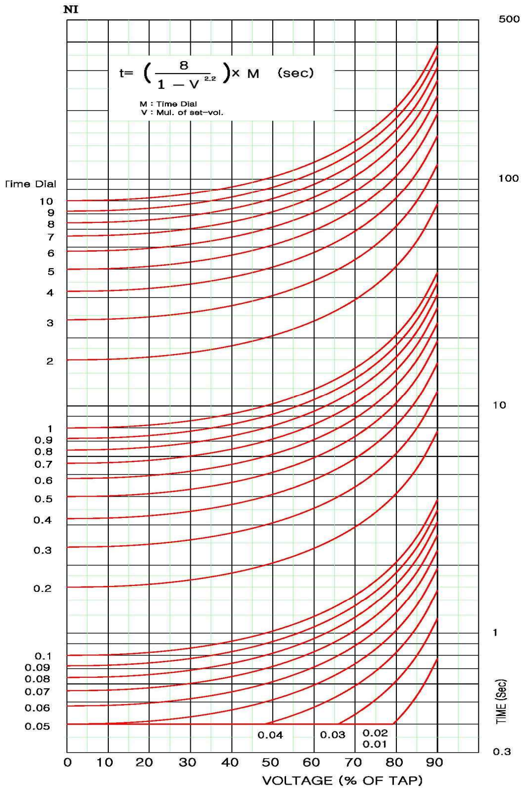
【부도 19】 저전압 역반한시 특성 곡선
