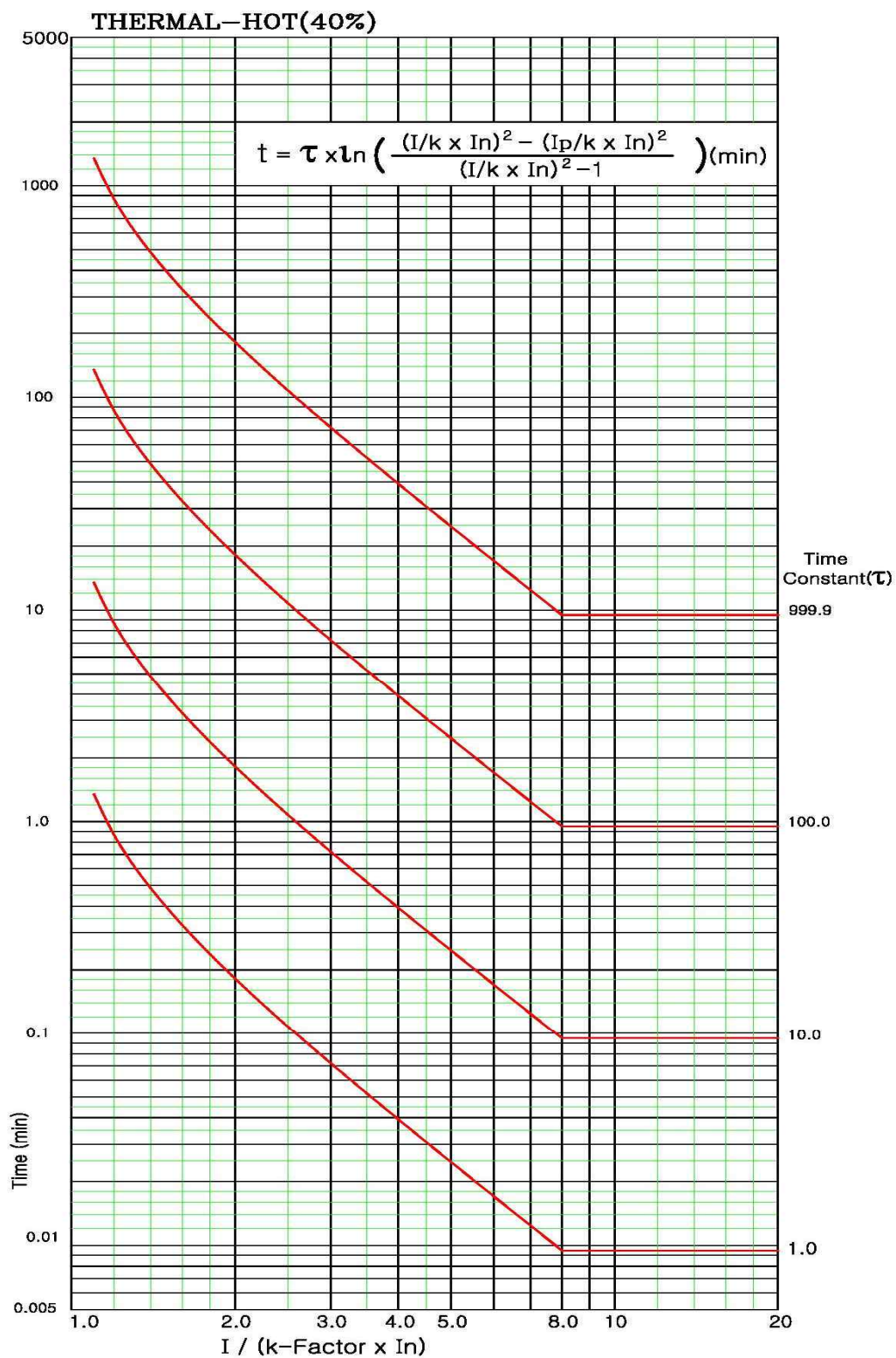
【부도 23】 THERMAL HOT 상태 특성 곡선
