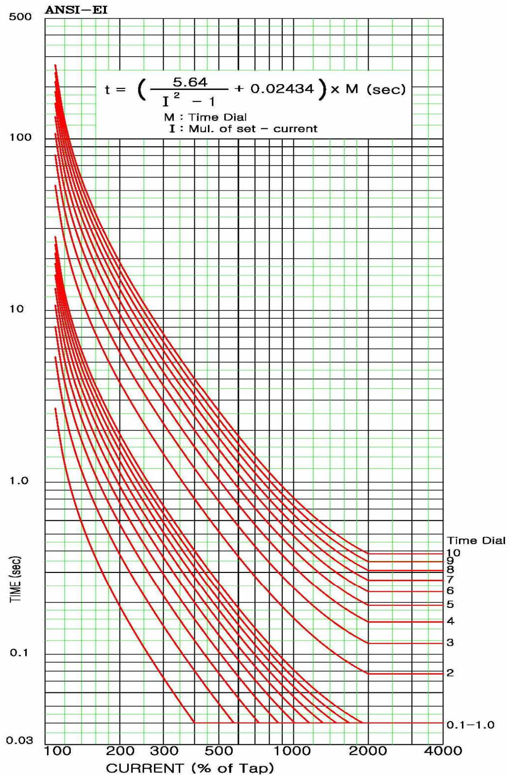
【부도 12】 과전류, 지락과전류, 역상과전류 ANSI_EI 특성 곡선
