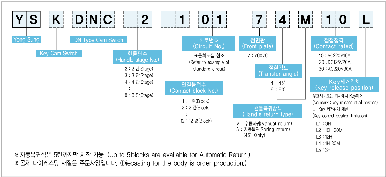
형식 구분도 | Type Classification Diagram - KDNC |
