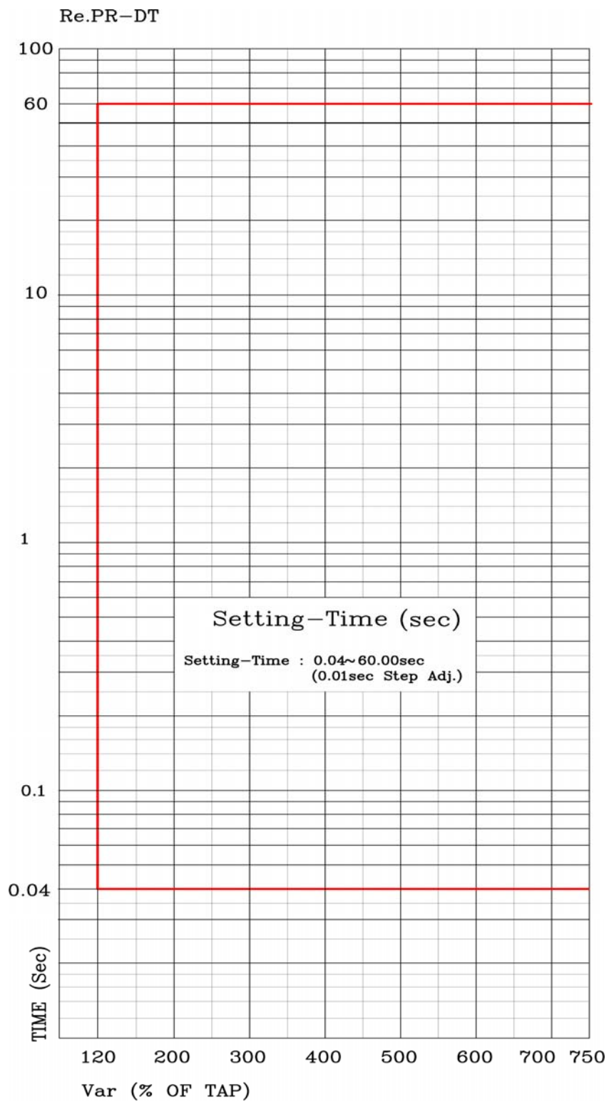
【부도 10】 무효전력 요소 정한시 특성 곡선
