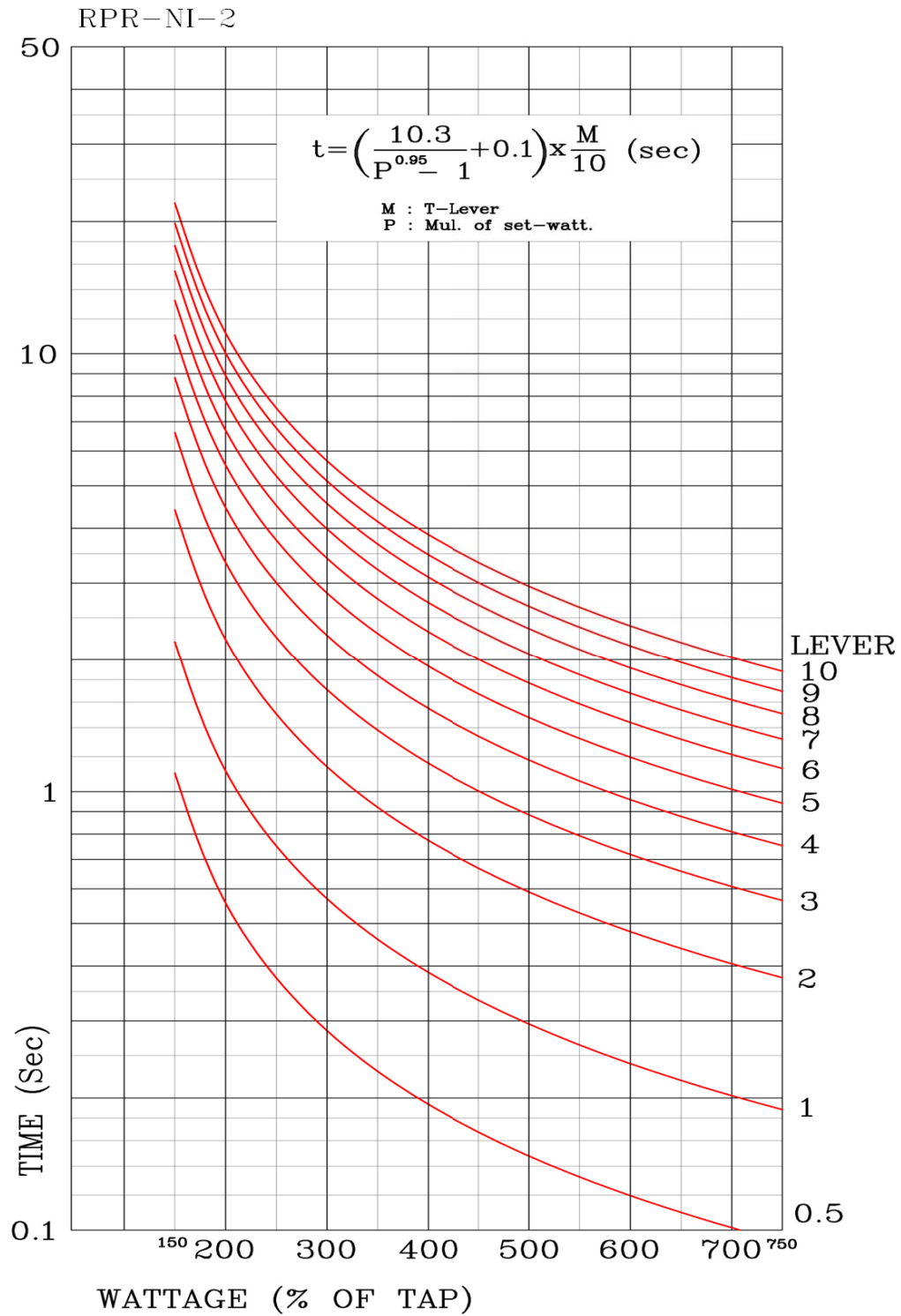
【부도 5】 역전력 요소 반한시 특성 곡선
