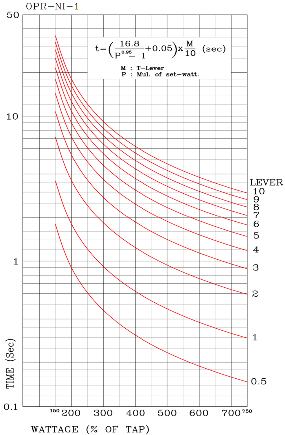
【부도 4】 과전력 요소 반한시 특성 곡선
