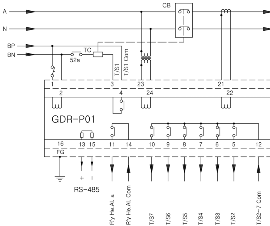
【부도 3】 외부 결선도
