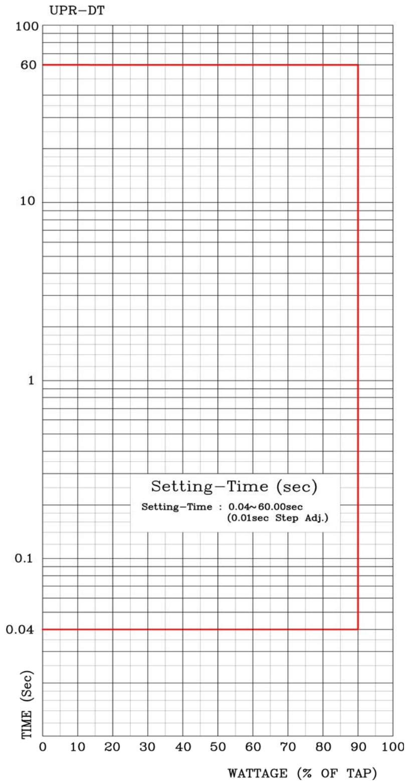
【부도 8】 저전력 요소 정한시 특성 곡선
