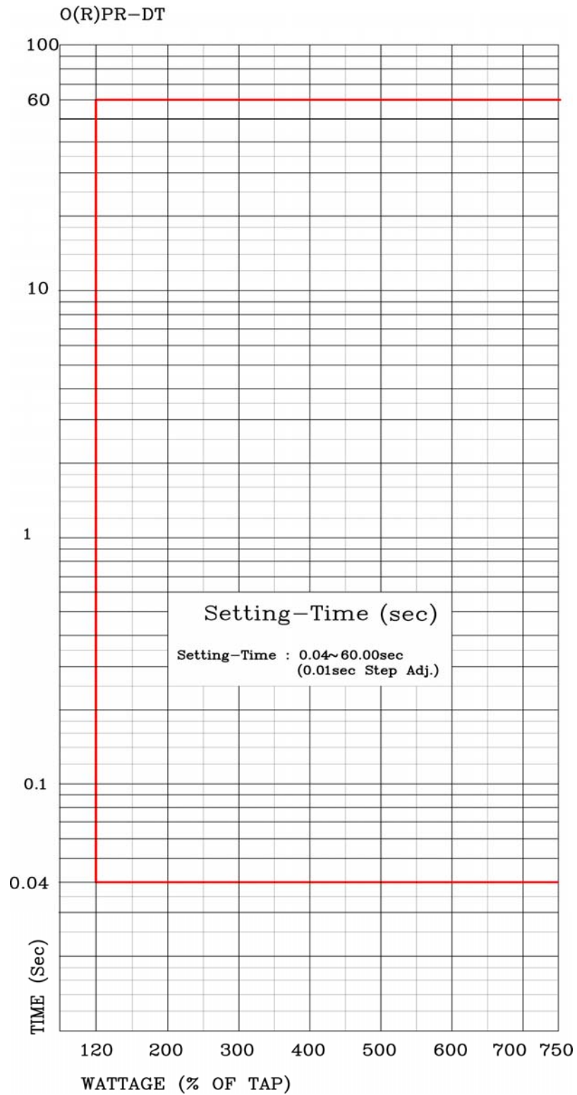
【부도 6】 과(역)전력 요소 정한시 특성 곡선
