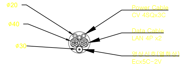
"A" CABLE 단면
