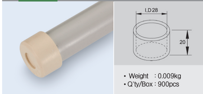
GAP-02B Plastic Joint ("D"부 관통)
