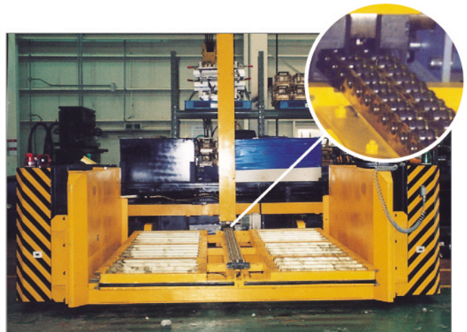
◀ 궤도식 사출기 금형교환대차 - 현대모비스 러시아공장 제작납품
