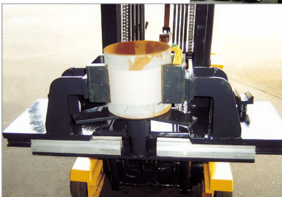
조선소 관통파이프 핸들링
