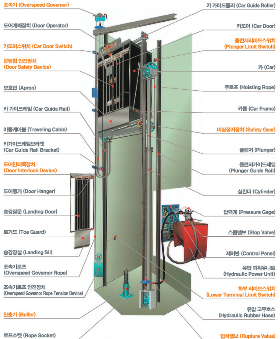
▲ 주황색으로 표기된 명칭은 승강기의 주요 안전장치입니다.
